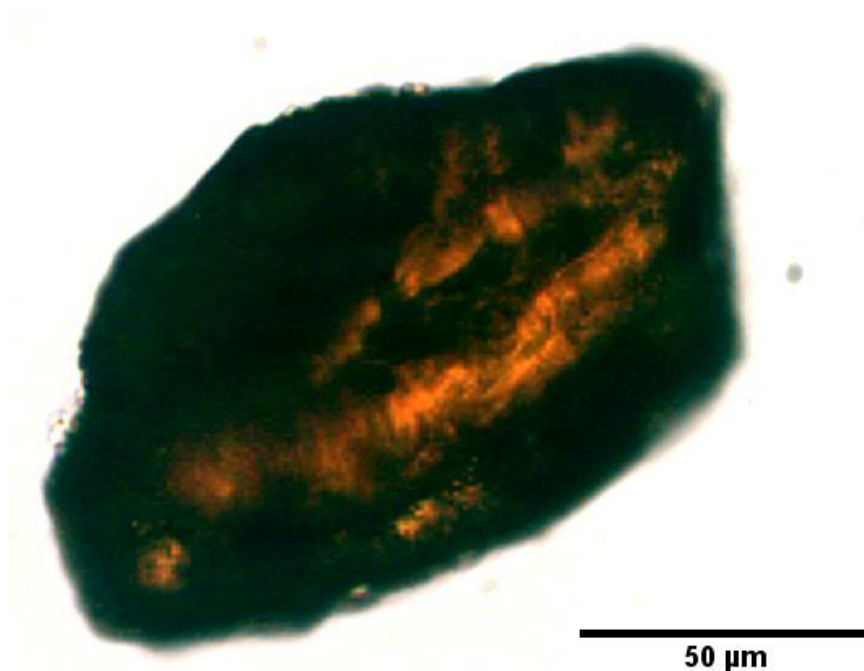
Slika 6-21. Zaobljeno zrno rutila, uzorak G-3.
