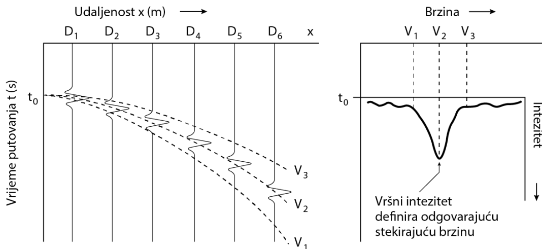
Slika 3-7 Skup tragova za istu CMP-točku koji će biti NMO korigirani koristeći raspon brzina. Stekirajuća brzina je ona za koju zbrojeni trag ima najveći intenzitet, odnosno amplitudu. U danom primjeru V_2 predstavlja stekirajuću brzinu. (Taner i Koehler, 1969)
