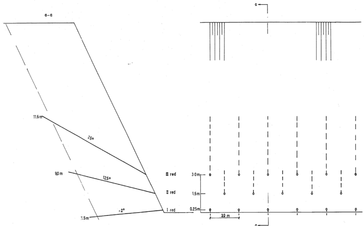
Slika 4-2 Shema bušenja dubokih minskih bušotina (Vrkljan i dr., 1993)
