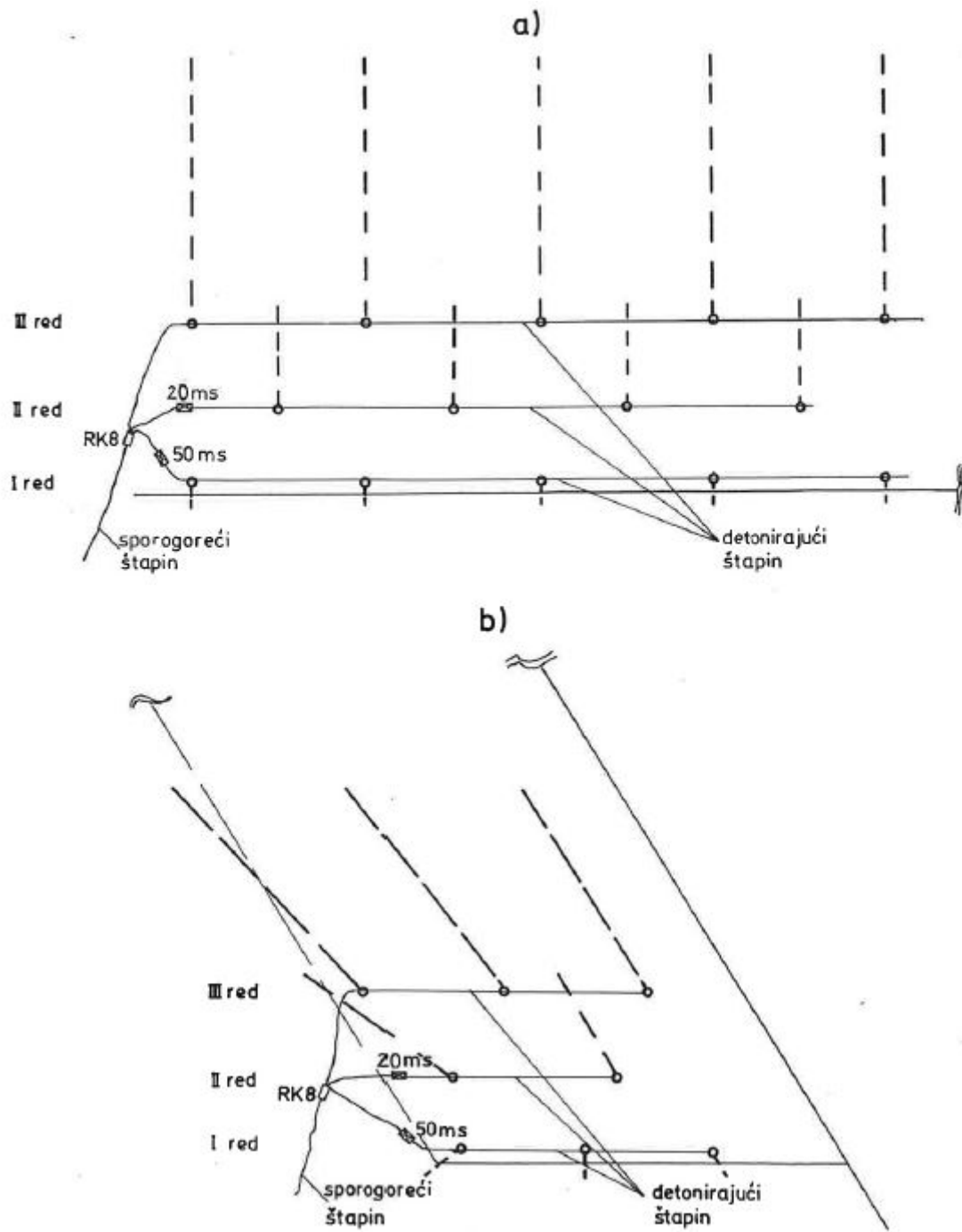
Slika 4-3 Sheme povezivanja usporjenja i paljenja minskog polja: a) frontalno, b) bočno (Vrkljan i dr., 1993)
