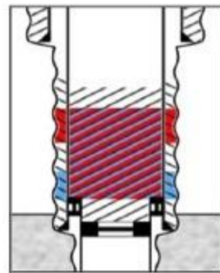
Slika 2. 4. Zajednička barijera: cementni čep (Norsok Standard D-010, 2013.)
