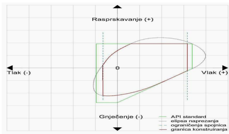
Slika 2. 2. Elipsa napreznja konstruiranja opreme (Norsok Standard D-010, 2013.)
