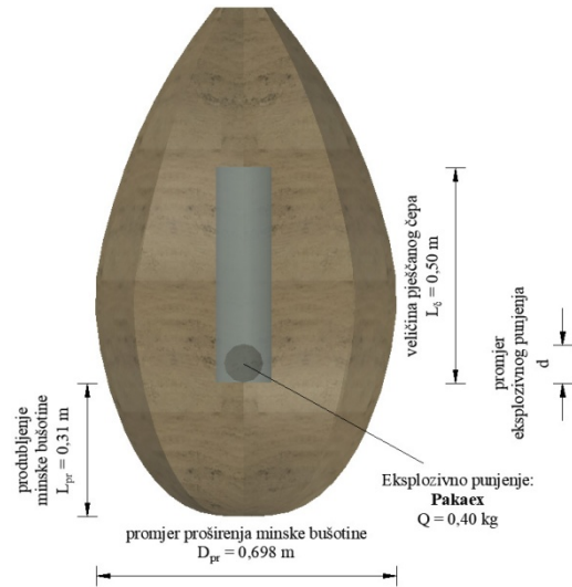
Slika 11.34 3D model nastalog proširenja minske bušotine MB 15, AutoCad Civil 3D
