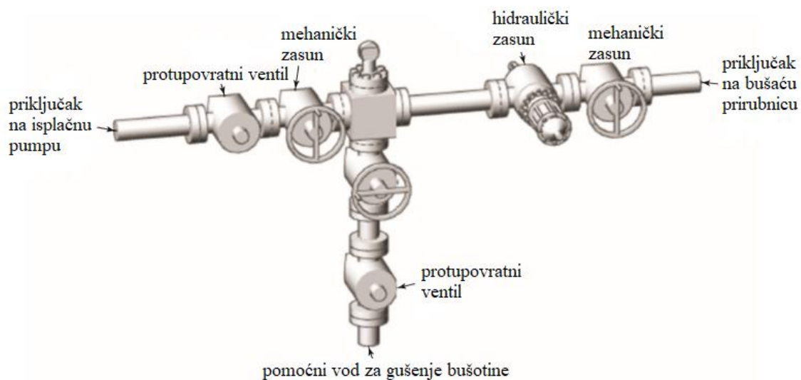
Slika 3-3. Vod za gušenje bušotine za radni tlak od 69 MPa (10 000 psi) ili više (API Specification 16C, 2015)
