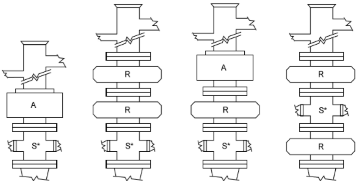
Slika 2-2. Konfiguracija preventerskog sklopa s bušaćom prirubnicom za radni tlak od 13,8 MPa (2 000 psi) (Well Control for the Rig-Site Drilling Team, 2002)
