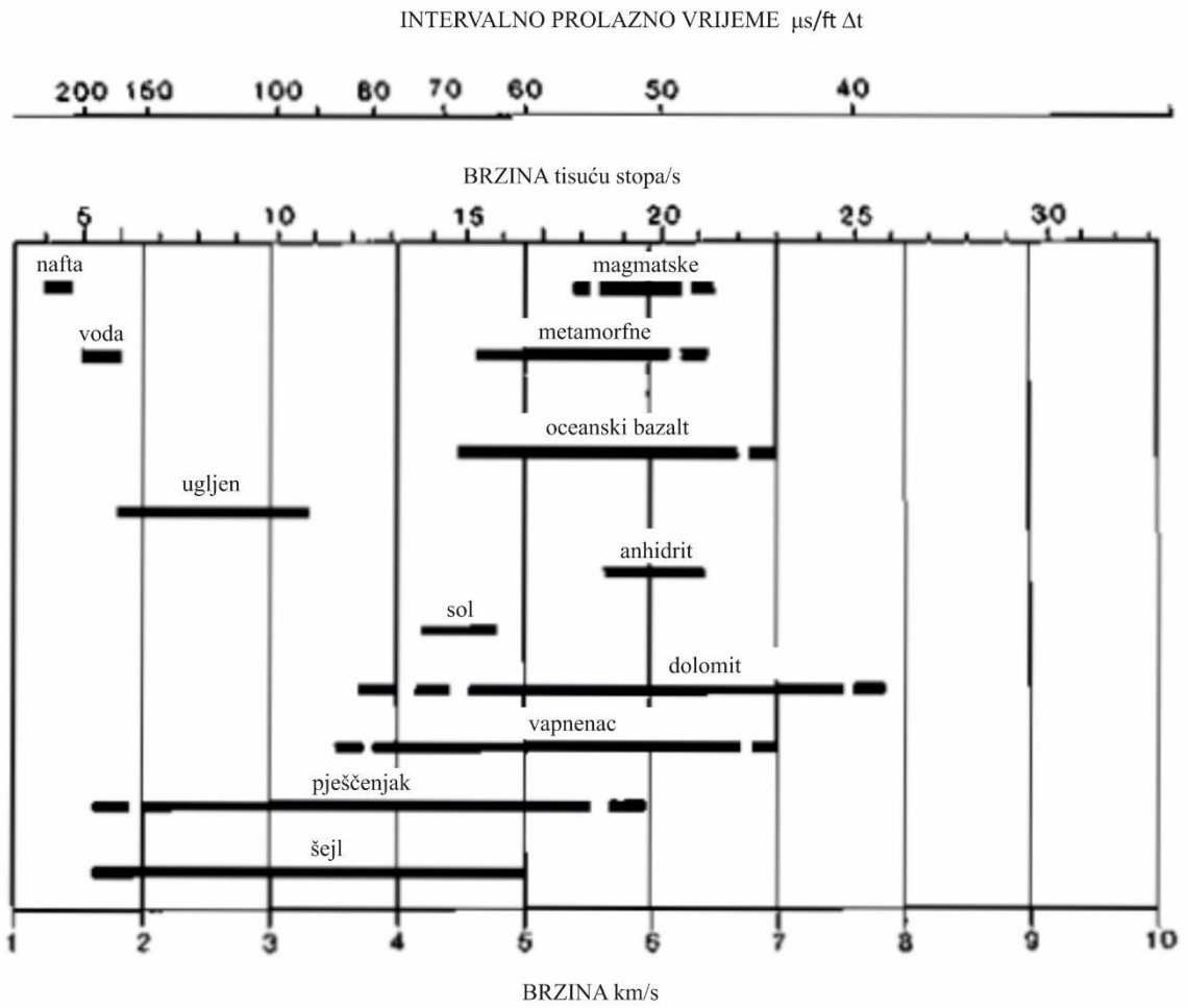
Slika 4-2. Prosječne brzine rasprostiranja valova u stijenkama (ft – oznaka za stopu, a ona iznosi 0,3048 m) (Rider, 1996)
