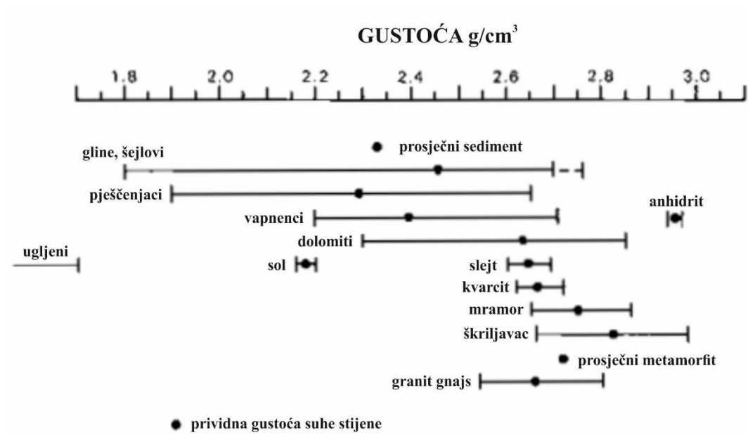
Slika 4-3. Rasponi gustoća stijena (Rider 1996 modificirano prema Jackson i Talbot, 1986)
