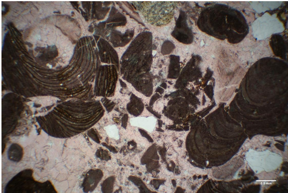
Slika 4-3. Mikropetrografski izbrusak, UZORAK BP-13 (paralelni nikoli) → biosparrrudit s bioklastima koralinacejskih algi te podređeno fragmentima ježinaca i česticama kvarca
