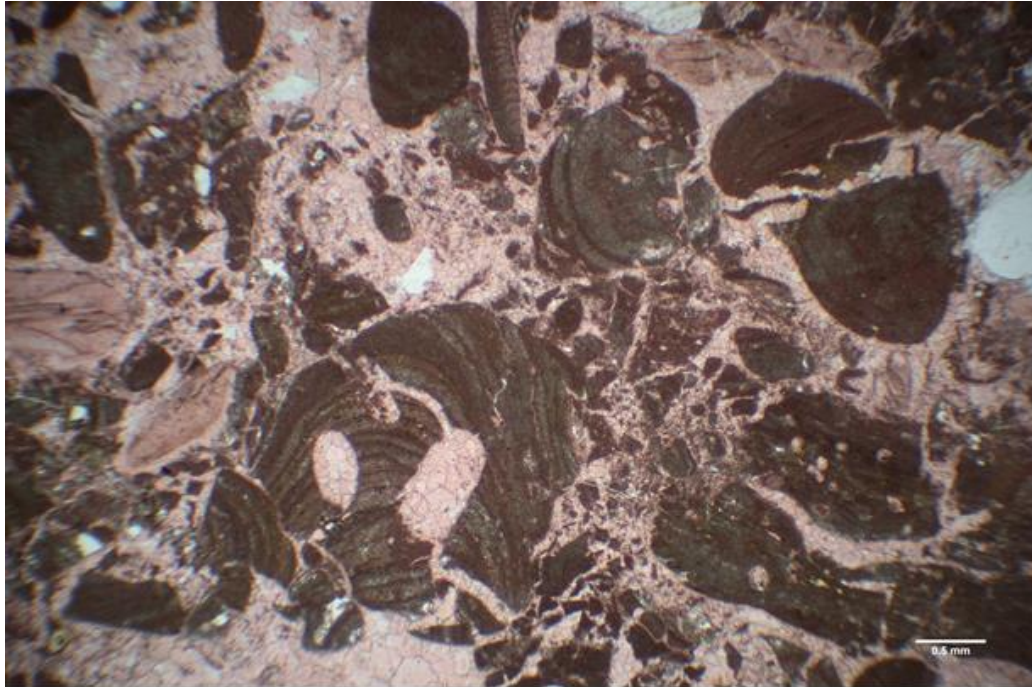
Slika 4-2. Mikropetrografski izbrusak, UZORAK BP-9 (paralelni nikoli) → biosparrrudit građen od bioklasta koralinacejskih algi i fragmenata ježinaca
