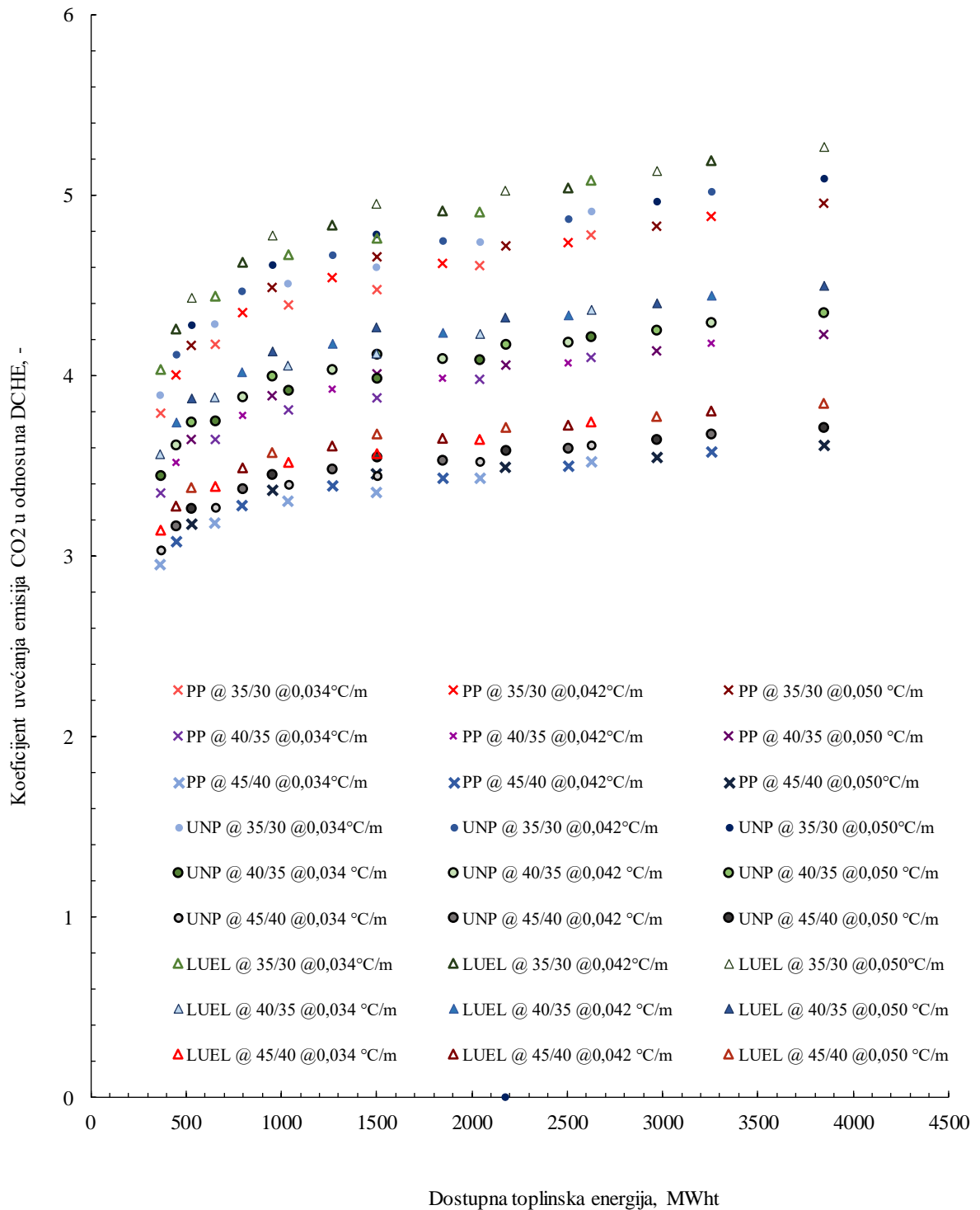
Slika 7.36. Koeficijenti emisija ugljikovog dioksida iskazani kao omjeri u odnosu na emisije proizašle korištenjem električne energije potrebne za rad dubokog bušotinskog izmjenjivača, na primjeru protoka od 15 l/s i različitim geotermalnim gradijentima
