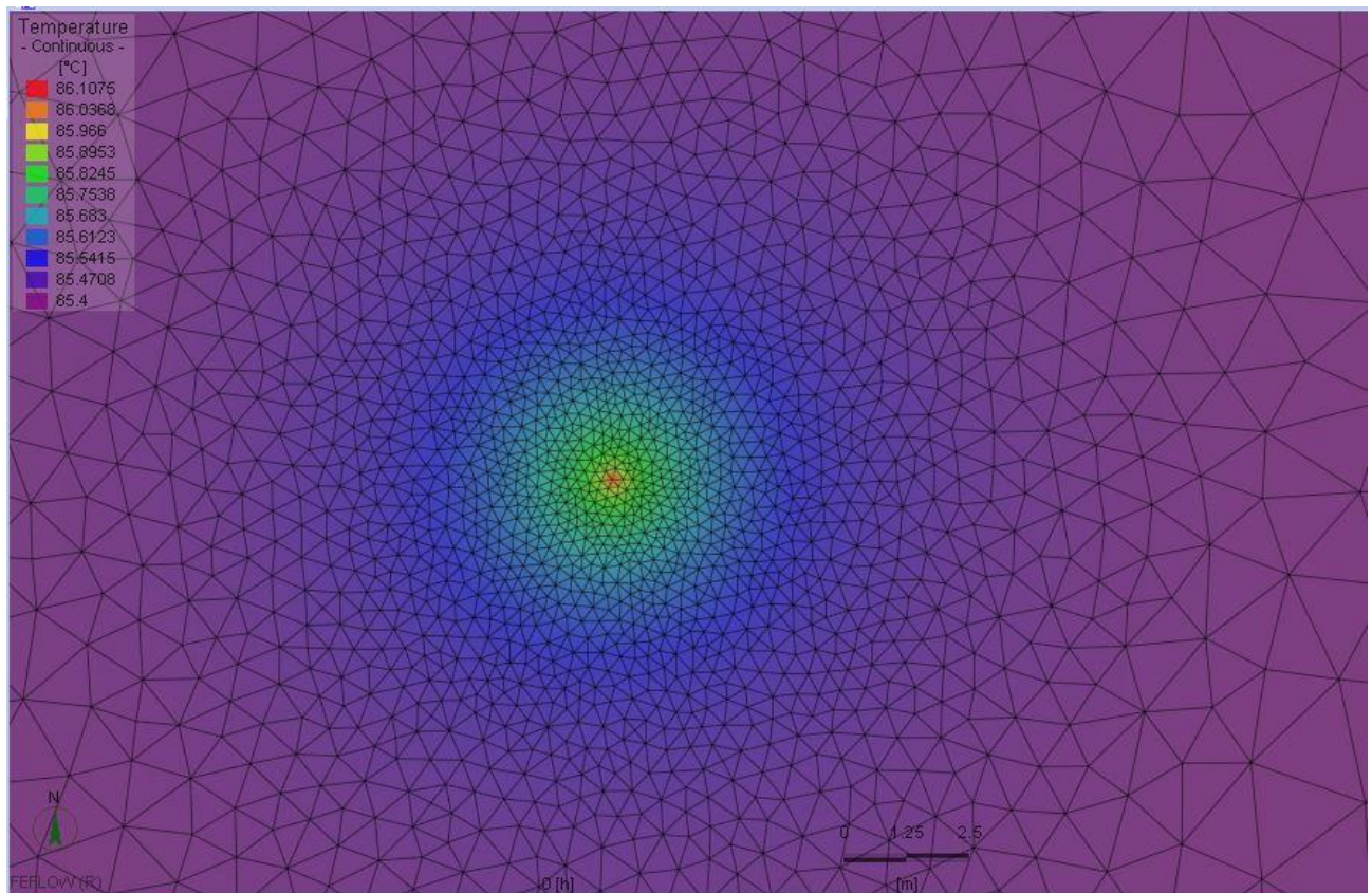
Slika 6.23. Prikaz širenja toplinske fronte na dubini 1800 m (slika zaslona)
