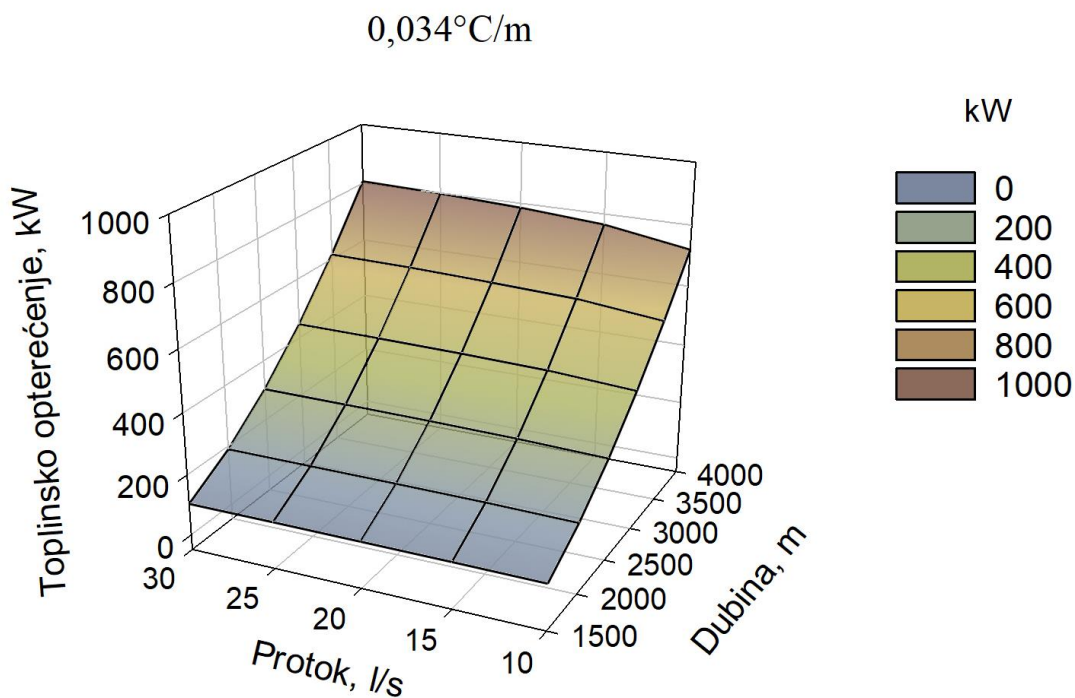
Slika 7.7. Rezultati dostupnih toplinskih opterećenja pri konstantnim toplinskim opterećenjima za temperaturni režim LST do 10 °C kod upotrebe izoliranog tubinga, pri geotermalnom gradijentu 0,034 °C/m za različite uvjete dubine i protoka
