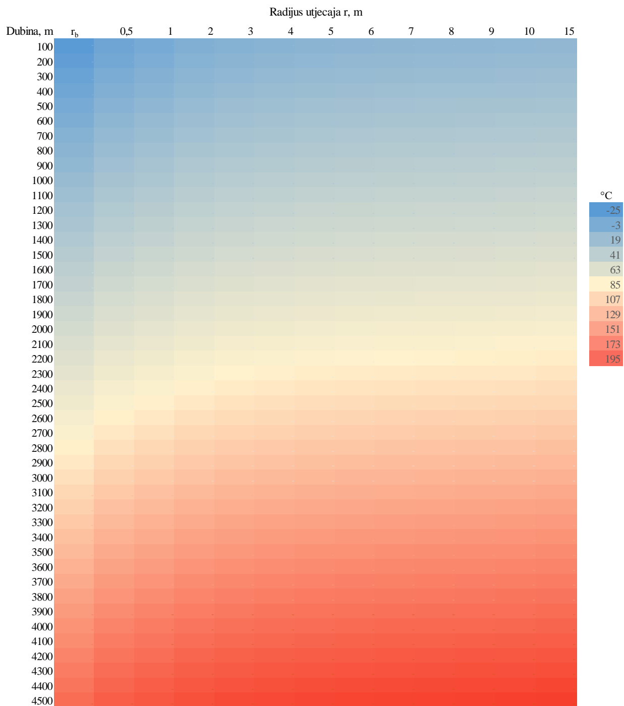
Slika 6.12. Promjena temperature za bušotinu Pčelić-1 prilikom konstantnog toplinskog opterećenja od 500 kW t u radijusu do 15 m.
