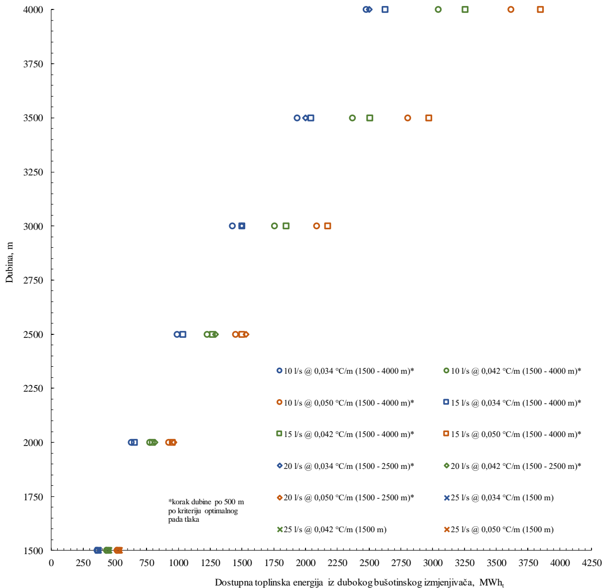
Slika 7.29. Dostupna toplinska energija za varijabilno toplinsko opterećenje za tri odabrana geotermalna gradijenta ( 0,034\text{ }^{\circ}\text{C/m} , 0,042\text{ }^{\circ}\text{C/m} i 0,050\text{ }^{\circ}\text{C/m} ), pri različitim protocima i dubinama bušotinskog izmjenjivača kod nižeg temperaturnog razreda
