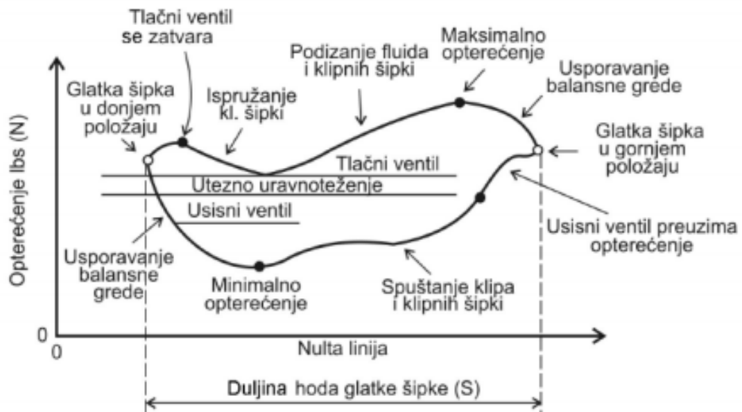
Slika 2-7. Dinamogram opterećenja klipnih šipki (Zelić i Čikeš, 2006)
