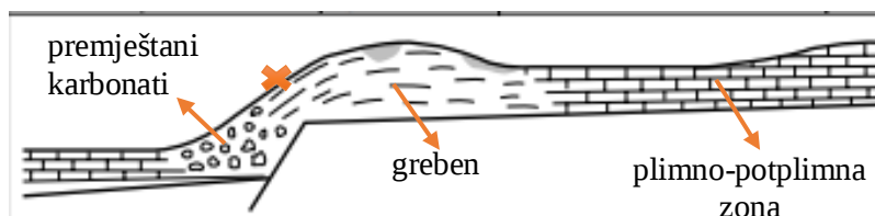
Slika 6-1. Mogući taložni okoliši istraženog područja (prilagođeno prema Tuckeru 2008); narančasti X označava najvjerojatniju poziciju taloženja istraživanih uzoraka
