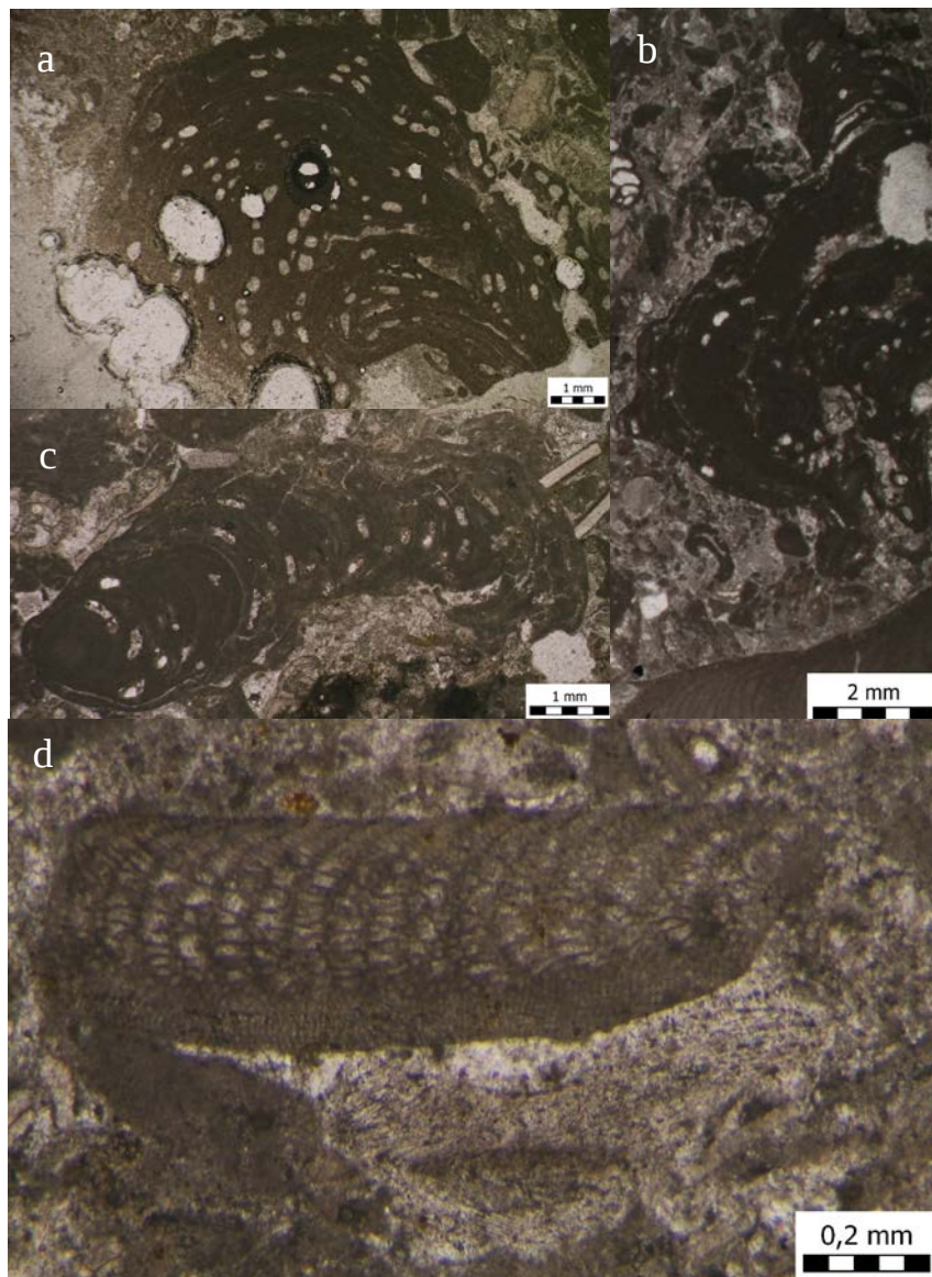
Slika 5-2. Determinirane crvene alge: a) i b) korasti oblici vrste Mesophyllum roveretoi ; c) prstasti oblik vrste Lithotamnion valens ; d) longitudinalni presjek vrste Subterraneanophyllum thomasi
