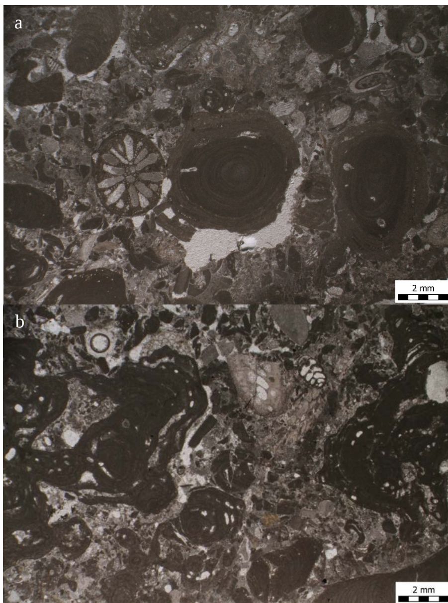
Slika 5-8. Floutstoni: a) Rodolitno-briozojski floutston; b) Koralinacejski floutston
