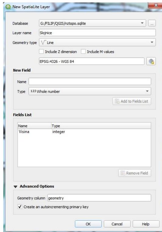
Slika 3-2 Stvaranje New SpatialLite Layera
