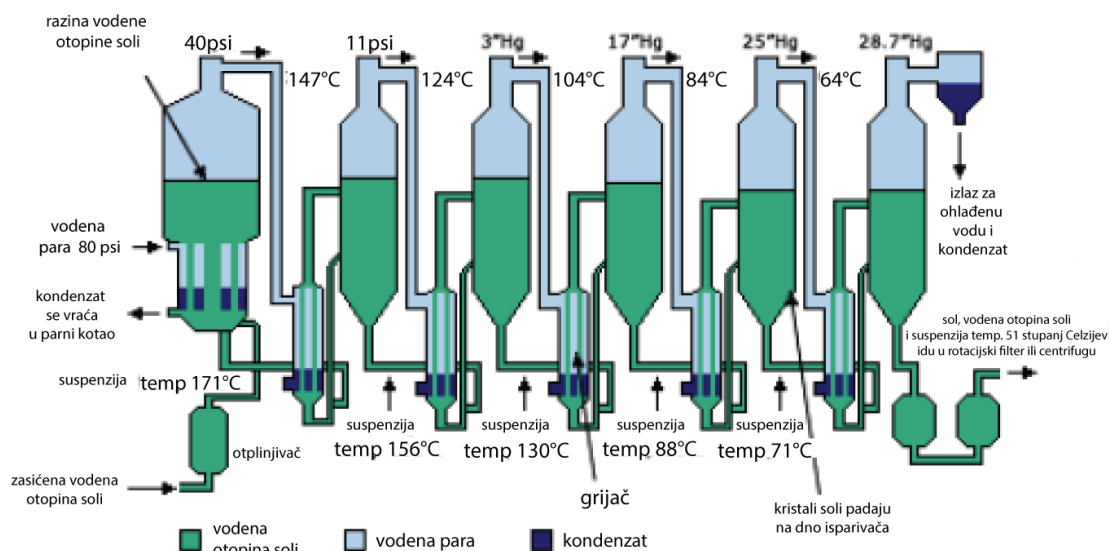
Slika 6-1. Postrojenje za preradu soli vakuumom (Eu-China Energy and Environment Programme, 2009)
