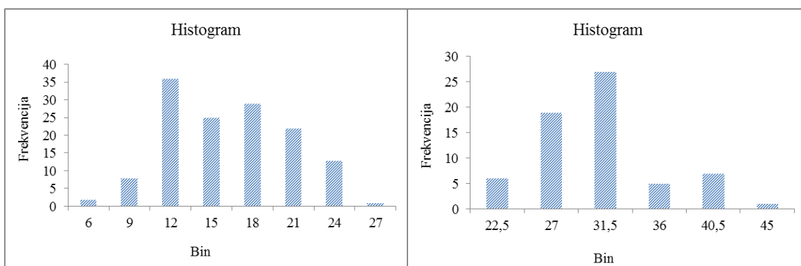
Slika 5.4. Razdioba podataka s postaja 941 (lijevo) i 5243 (desno)
