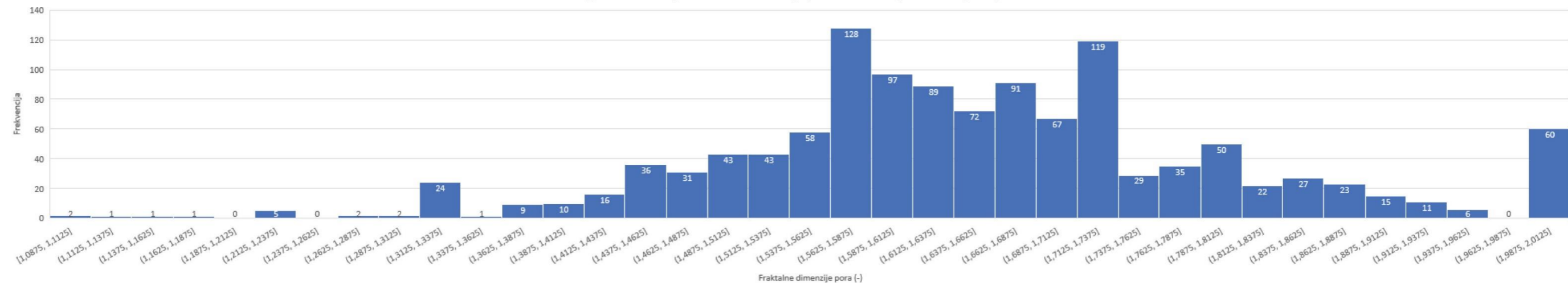
Prilog 1-3. Histogrami frekvencija AR-a, Feret AR-a i fraktalnih dimenzija pora člana Vranjak formacije Slapnica.
