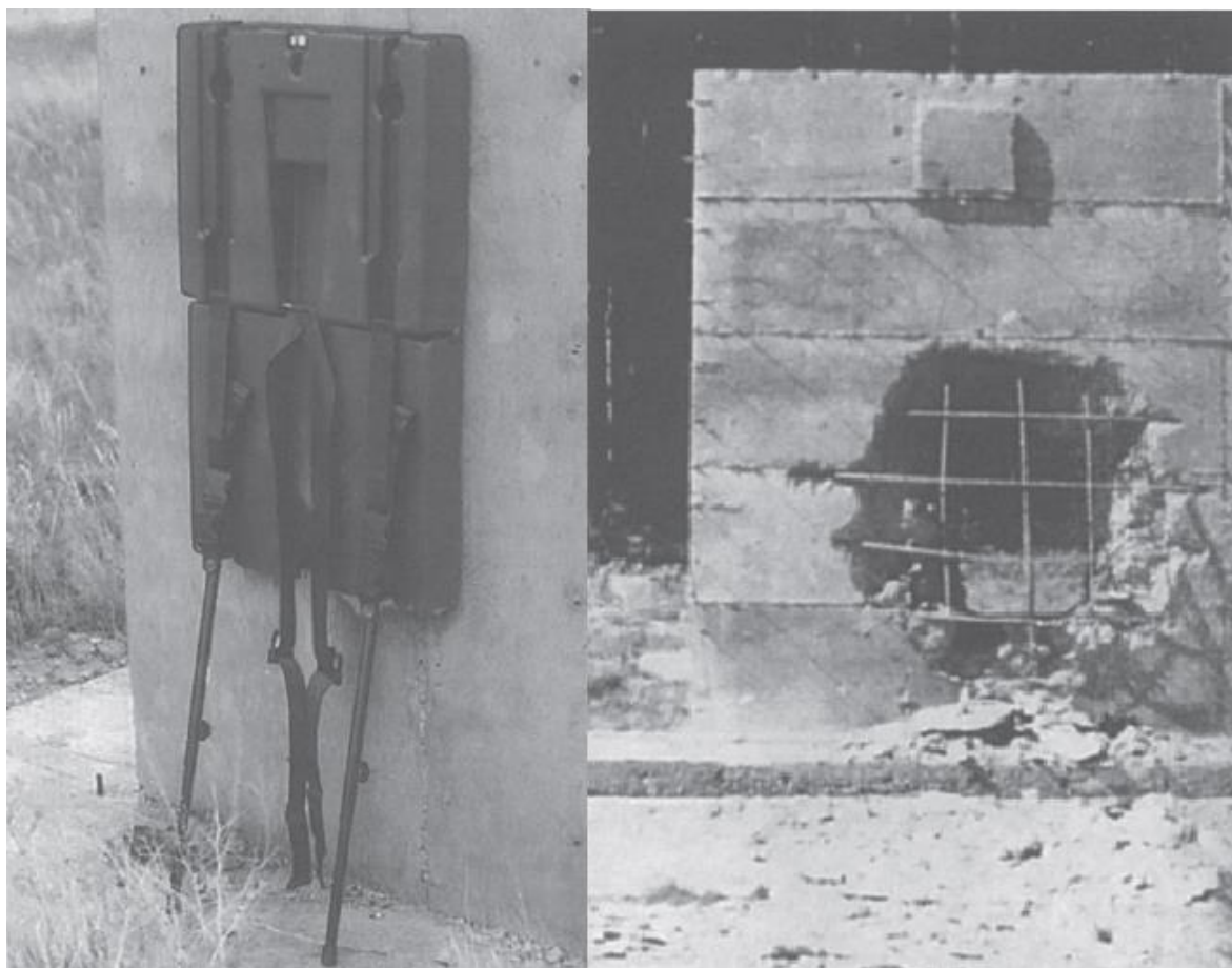
Slika 6-24 Primjer uređaja za razbijanje zidova "Breachcase" za vojne primjene (slika lijevo) i rezultati njegovog djelovanja (slika desno) (Weickert, 1998)
