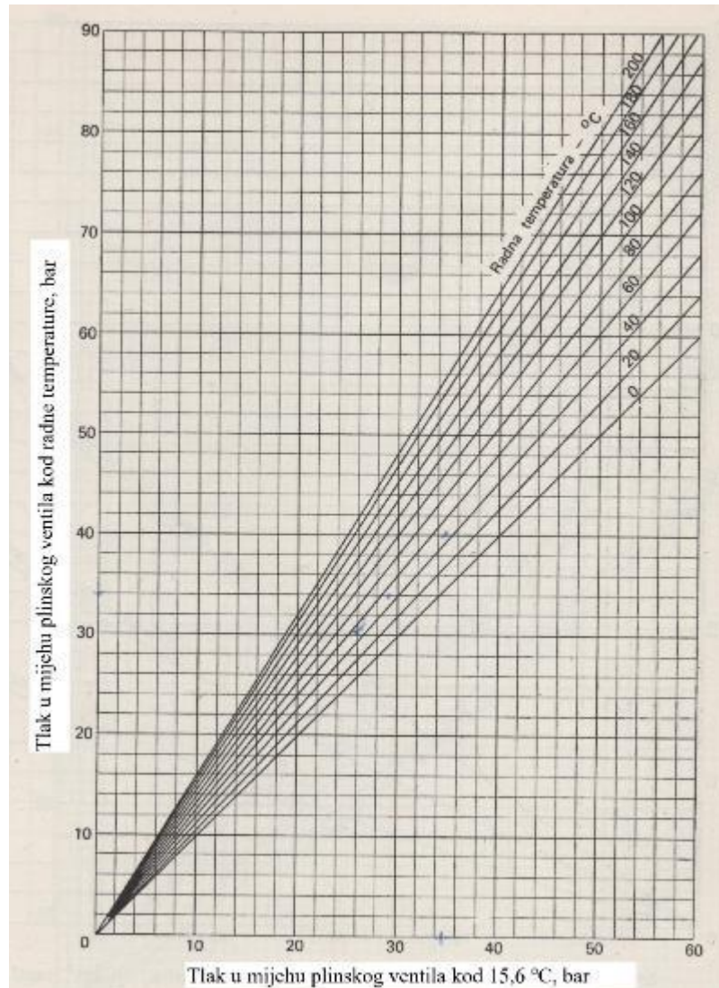
Slika 4-2. Dijagram ovisnosti tlaka u mijehu plinskog ventila pri radnoj temperaturi o tlaku pri standardnoj temperaturi (Zelić, 1977)
