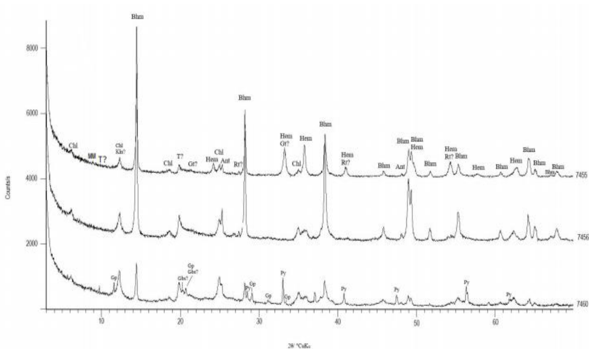
Slika 7.13. Difrakcijska slika jurskih boksita, Bm- bemit, Chl- klorit, Hem- hematit, MM- montmorilonit, Rt- rutil, Ant- anatas, T- titanit, Gt- getit, Py- pirit, Gbs- gibbsit, Gp- gips
