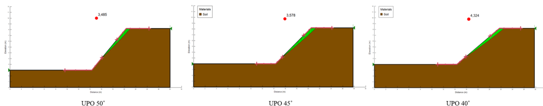
Slika 5.1. Prikaz rezultata proračuna stabilnosti kosine pri iskopu temeljnog tla.
