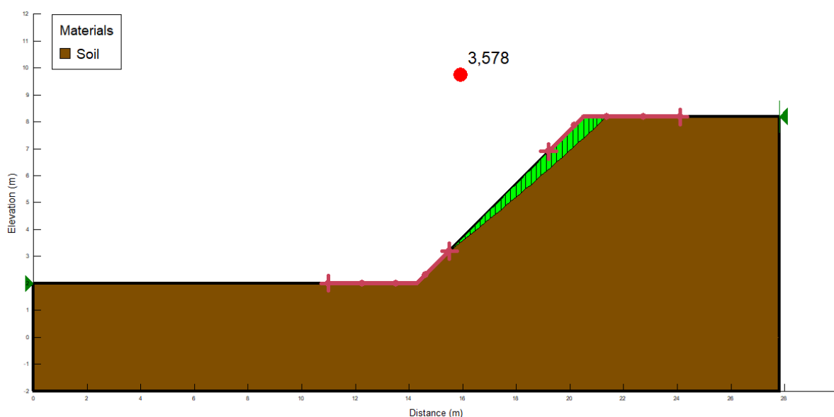
Slika 4.29. Kritična klizna ploha i faktor sigurnosti za kosinu nagiba 45^\circ pri iskopu temeljnog tla.
