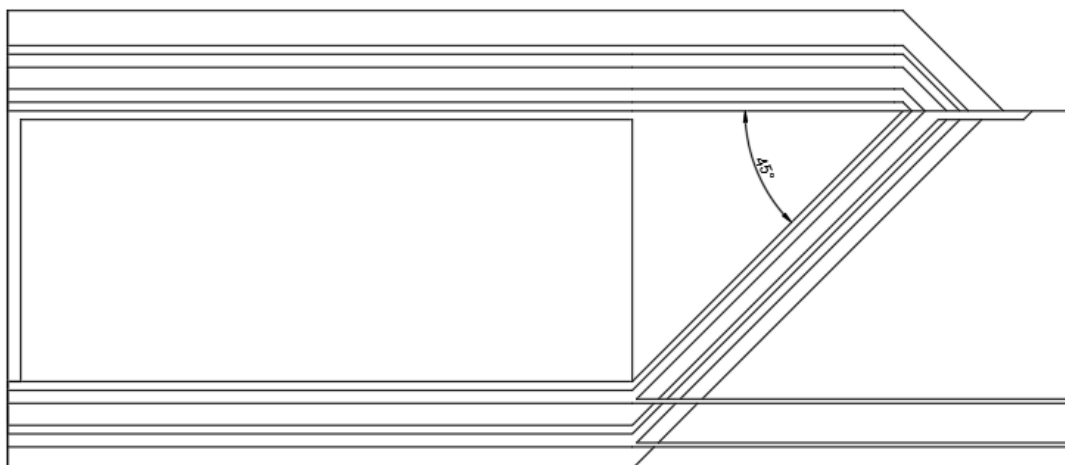
Slika 4.28. Nacrt simetričnog presjeka UPO s kutom nagiba 50^\circ .
