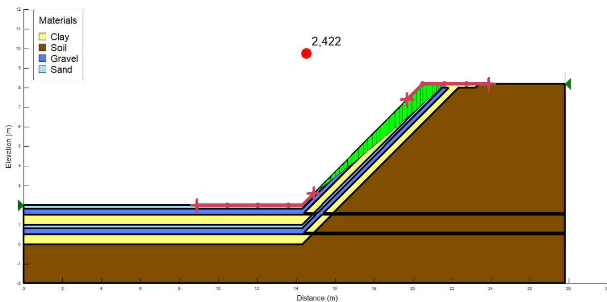
Slika 4.33. Kritična klizna ploha s faktorom sigurnosti, druga faza UPO s kutom nagiba 45^\circ .
