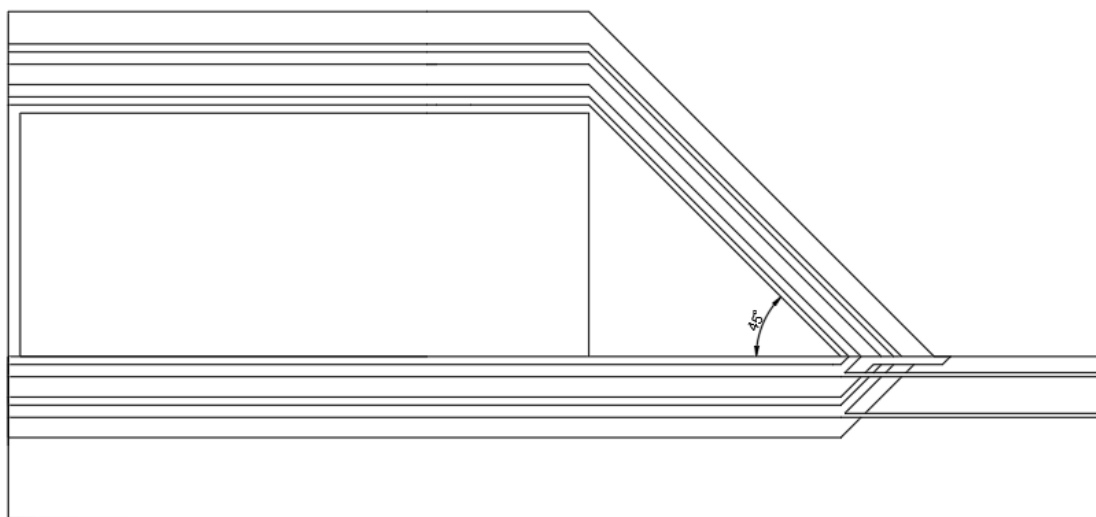
Slika 4.12. Nacrt simetričnog presjeka PPO s kutom nagiba 45°.
