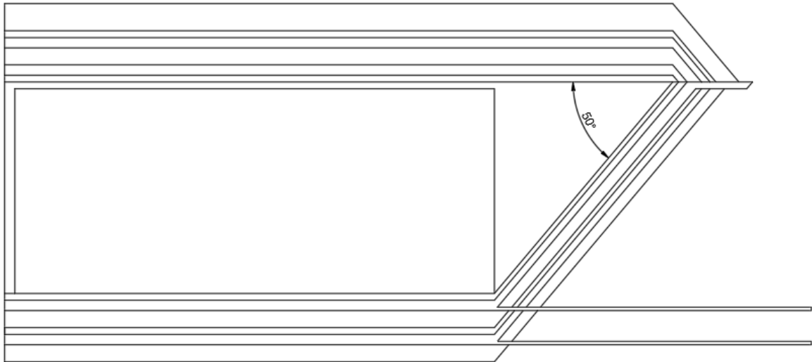
Slika 4.22. Nacrt simetričnog presjeka UPO s kutom nagiba 50^\circ .
