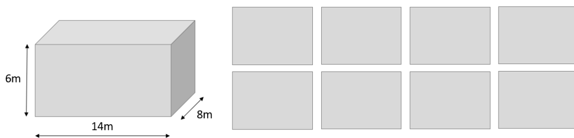
Slika 3.2. Dimenzija betonske kasete i pogled na raspored kaseti odozgo.
