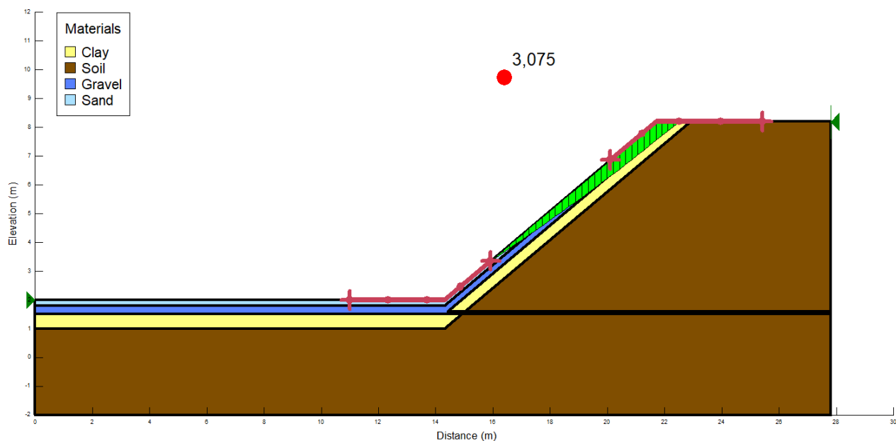
Slika 4.36. Krićna klizna ploha s faktorom sigurnosti, prva faza UPO s kutom nagiba 40^\circ .
