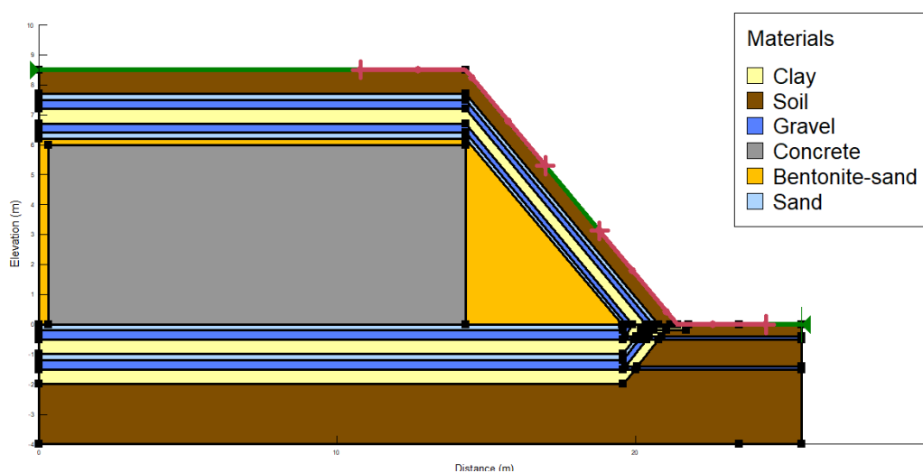
Slika 4.10. Druga faza PPO s kutom nagiba 50^\circ i Entry-Exit intervali.
