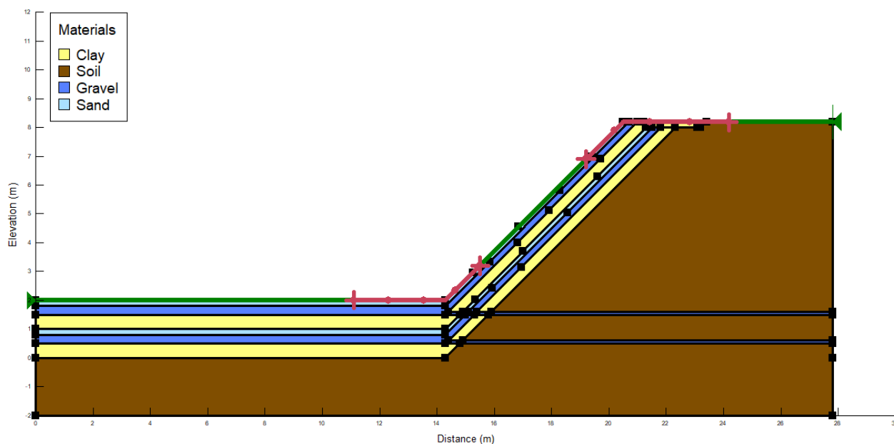
Slika 4.32. Druga faza UPO s kutom nagiba 45^\circ i Entry-Exit intervali.
