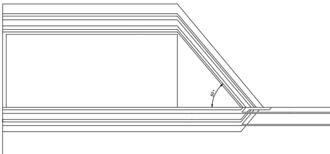
Slika 4.9. Nacrt simetričnog presjeka PPO s kutom nagiba 50^\circ .
