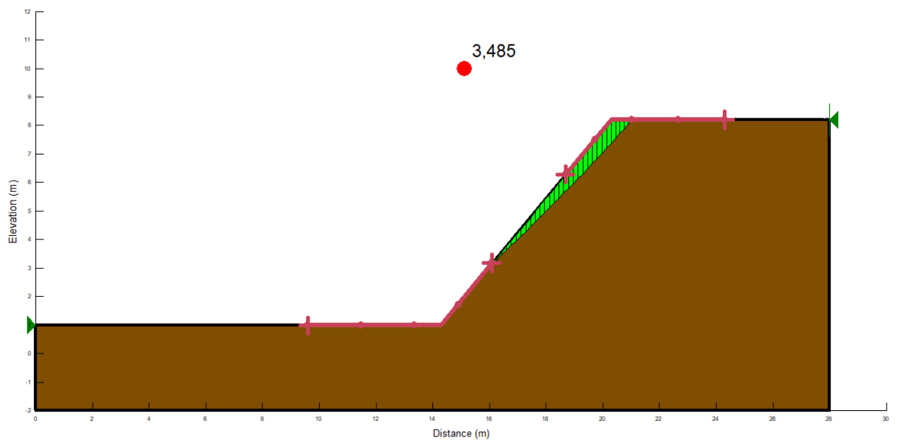
Slika 4.23. Kritična klizna ploha i faktor sigurnosti za kosinu nagiba 50^\circ pri iskopu temeljnog tla.
