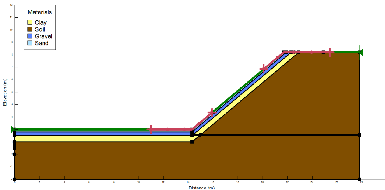
Slika 4.35. Prva faza UPO s kutom nagiba 40^\circ i Entry-Exit intervali.
