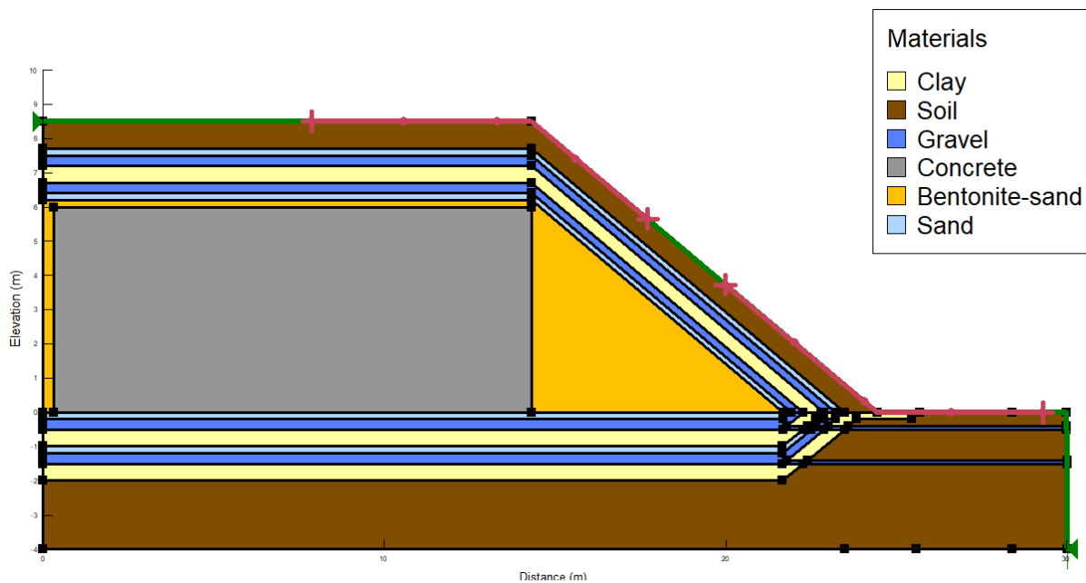
Slika 4.20. Druga faza PPO s kutom nagiba 40° i Entry-Exit intervali.
