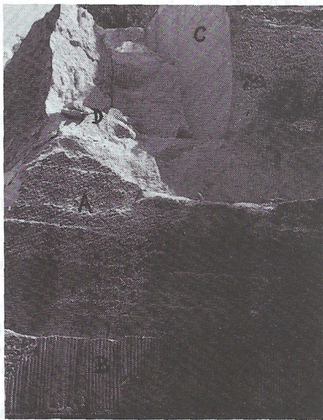
Sl. 18. Kamenolom na otoku Vrniku. Površinski kop visinskog tipa s ostacima četiri metode dobivanja blokova kamena: (A) stijenke pašarina iz antike s vidljivim strijama od rada dlijetom, (B) stijenke s tragovima gusto izbušenih rupa duž visine odvaljenog bloka, (C) rez helikoidalnom žičnom pilom i (D) raspucani i rastreseni vapnenac od djelovanja eksploziva rabljenog za odvajane nepravilnog bloka kamena. Rad pod (D) najnovijeg je datuma i za njega nema komentara (foto: D. Jovičić, 1996)
