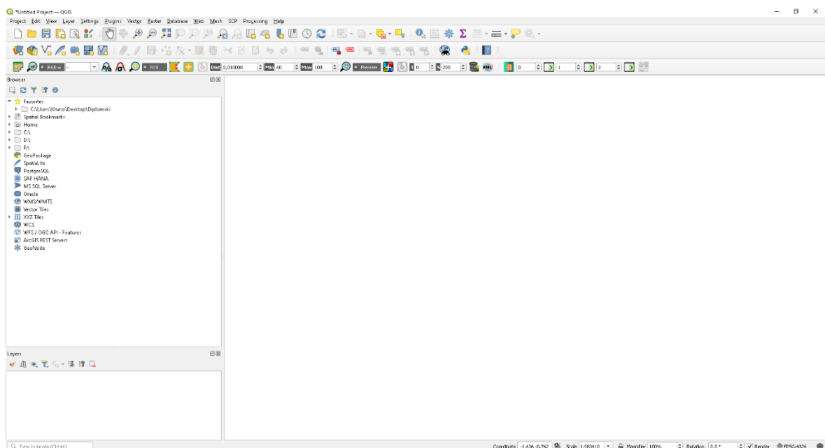
Slika 6-1 Sučelje QGIS-a
