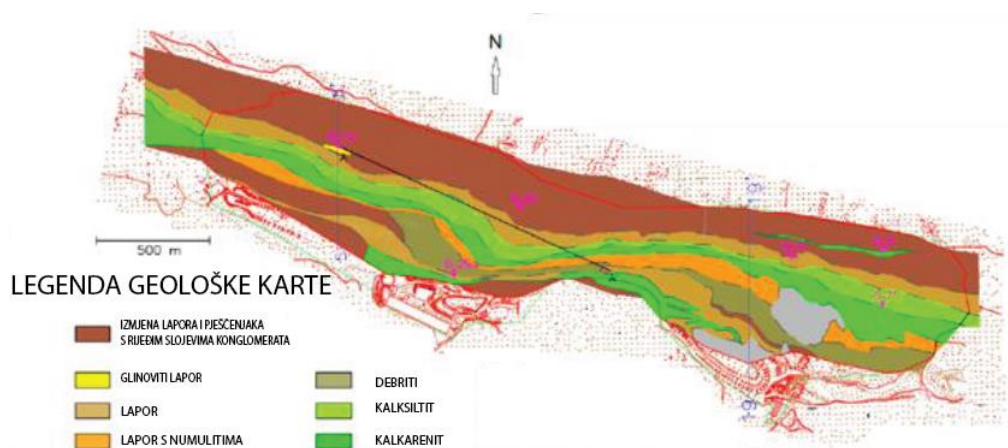
Slika 5-1. Geološka karta eksploatacijskog polja „Sv. Juraj – Sv. Kajo“ (Bralić i Malvić, 2022)
