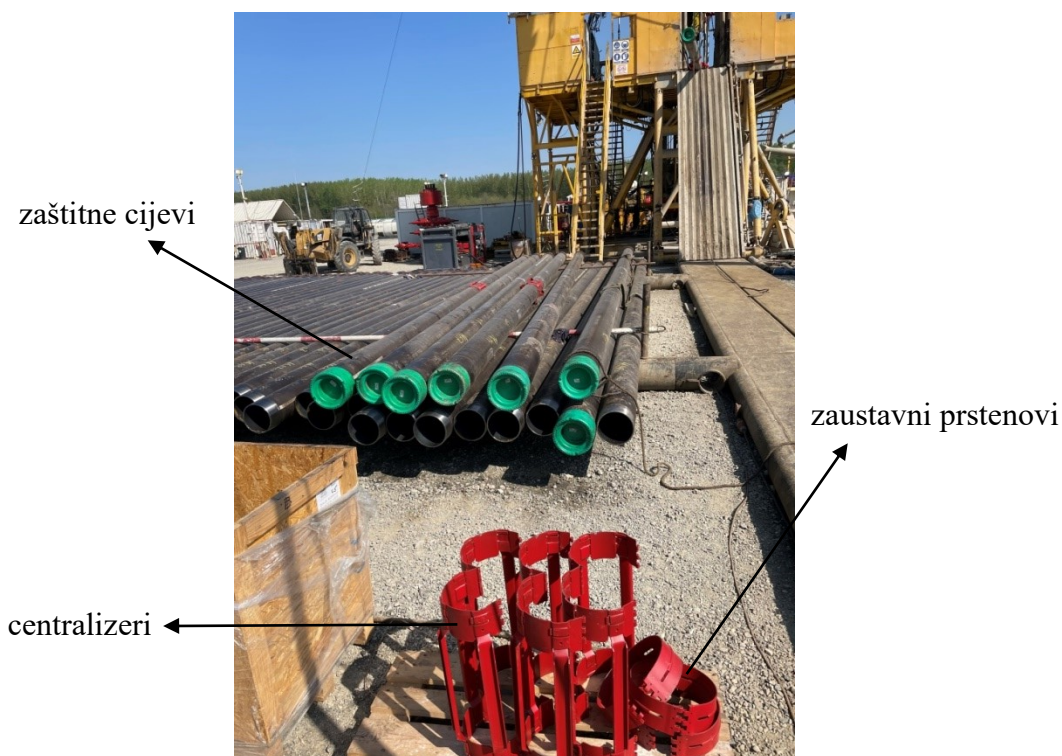
Slika 3-1. Centralizeri i zaštitne cijevi vanjskog promjera 0,2445 m (9 5/8")
