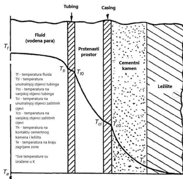
Slika 2-4. Distribucija temperature unutar bušotine (Ameli et al., 2018)
