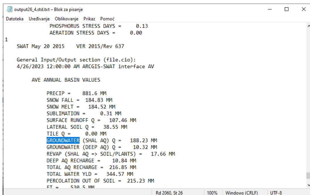
Slika 5-29. Output.std datoteka
