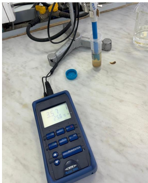
Slika 6-4. Mjerenje pH.
