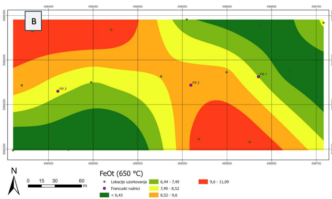
Slika 8-5. A) Karta interpolacije koncentracije FeOt(%) nakon zagrijavanja na 105°C; B) Karta interpolacije koncentracije FeOt(%) nakon zagrijavanja na 650°C (izrađeno u ArcGIS-u).
