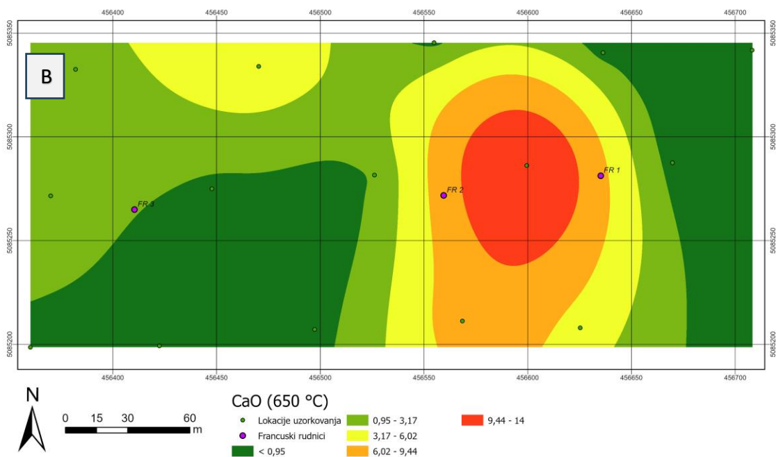
Slika 8-7 A) Karta interpolacije koncentracije CaO(%) nakon zagrijavanja na 105°C; B) Karta interpolacije koncentracije CaO(%) nakon zagrijavanja na 650°C.
