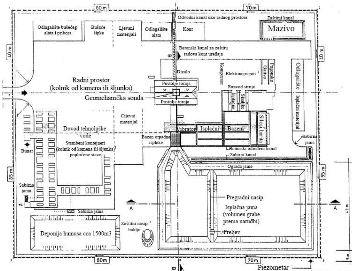
Slika 4-5. Shematski prikaz položaja isplačne jame na prostoru bušotine prema Glavnom tipskom rudarskom projektu (Rukavina et al., 1990)
