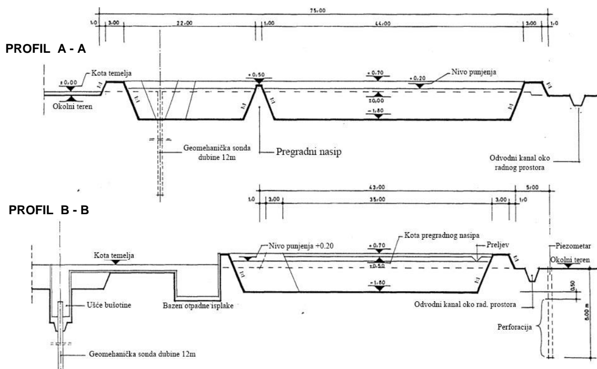
Slika 4-6. Presjeci isplačne jame s položajem piezometara i sonde (Rukavina et al., 1990)
