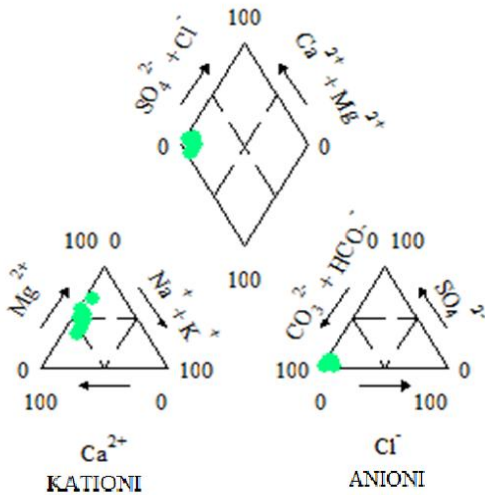
Slika 4.5. Piperov dijagram vodocrpilišta Topolje
