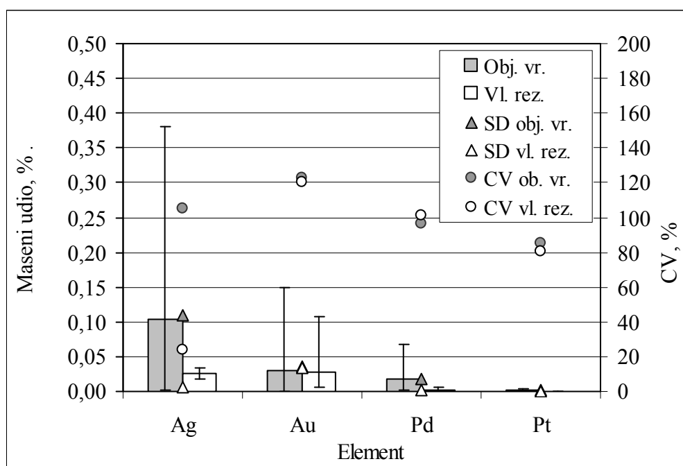
Slika 55. Prosječni maseni udio plemenitih metala u metalu u uzorcima TP dobivenih u okviru ovog rada u odnosu na objavljene vrijednosti drugih autora
