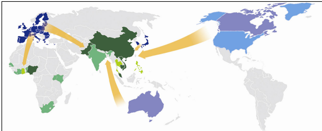
Slika 2 Svjetski tokovi EE otpada (Li et al., 2013)
