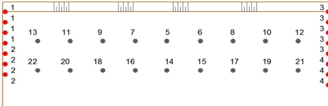
Slika 7-9. Redosljed otpucavanja minskih bušotina za I etažu
