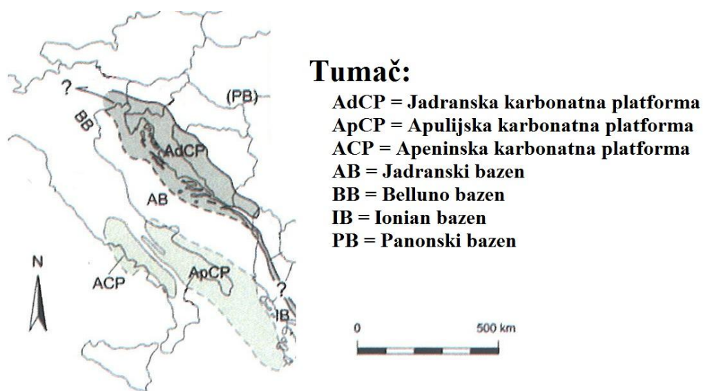
Slika 3.2. Područja prostiranja Jadranske, Apeninske i Apulijske karbonatne platforme (iz Vlahović et al., 2005, izmjenjeno). Na karti su prikazani i položaji dubokomorskih bazena koji su se otvorili između karbonatnih platformi.
