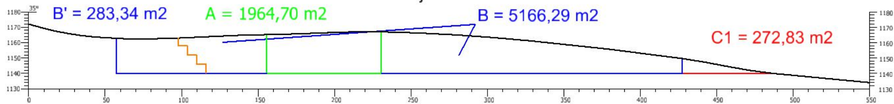
Presjek 7-7'
