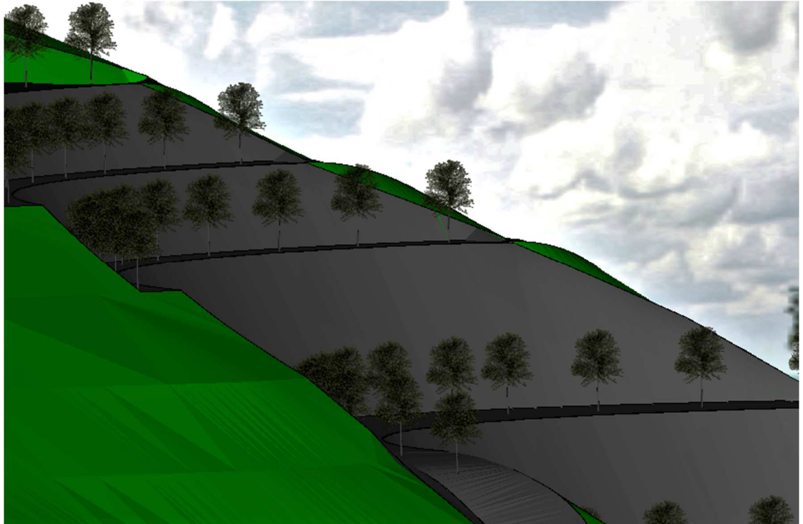
Slika 7-26. Sanirano stanje, gornji dio, pogled sa zapada
