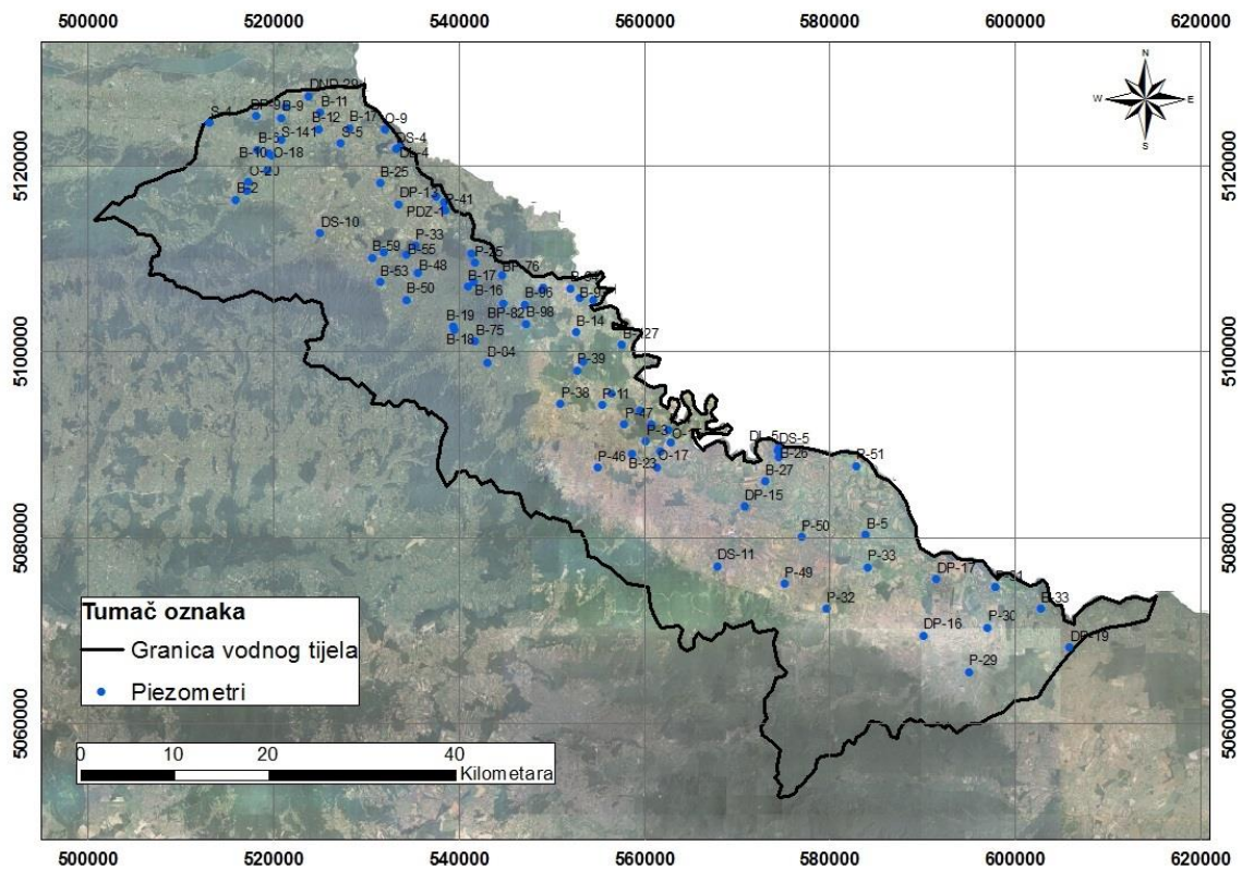
Slika 3-1. Prikaz piezometara na vodnom tijelu Legrad-Slatina
