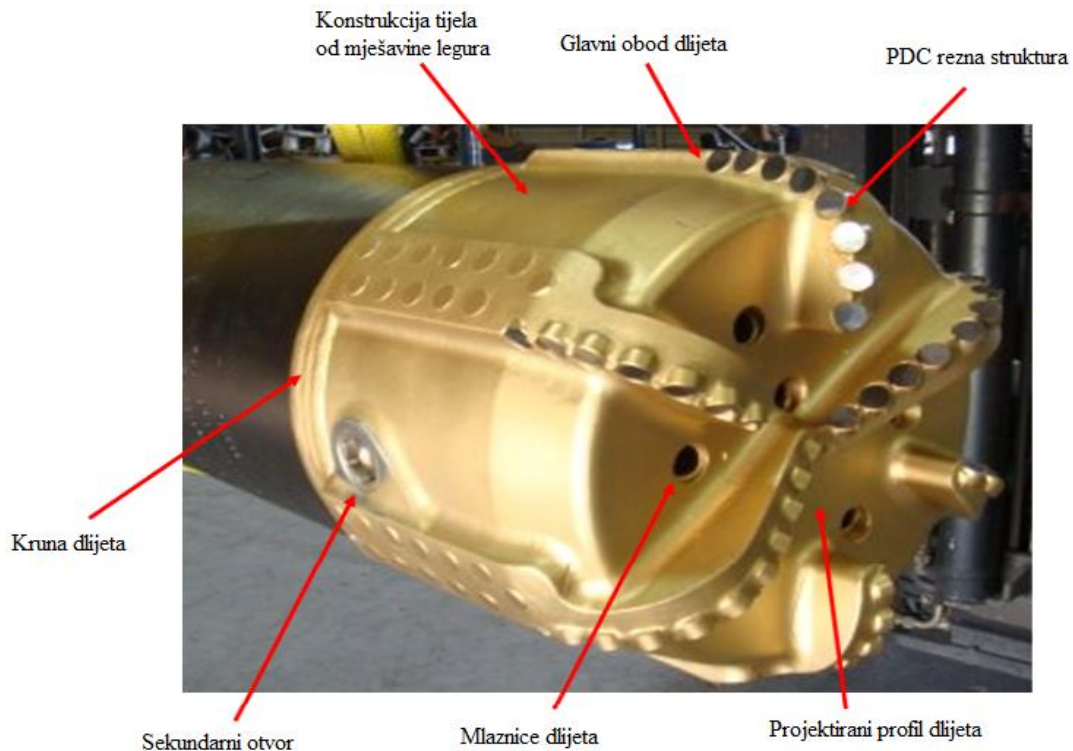
Slika 2-11. Dlijetno za bušenje uz primjenu lajnera od čelične figure sa šest oštrica (Kunning et al., 2009)
