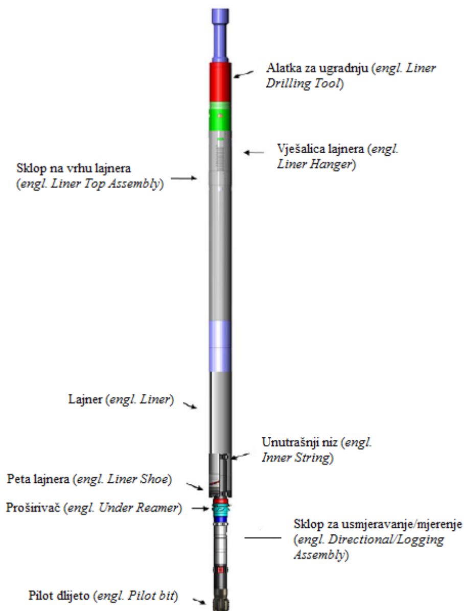
Slika 3-1. Sastav alata za bušenje uz primjenu lajnera i izvlačivog BHA (Eriksen et al., 2011)
