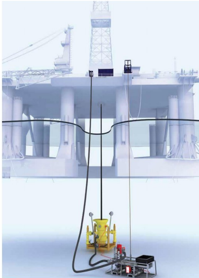
Slika 4-11. Metoda povrata isplake bez rajzer cijevi (www.enhanced-drilling.com).
