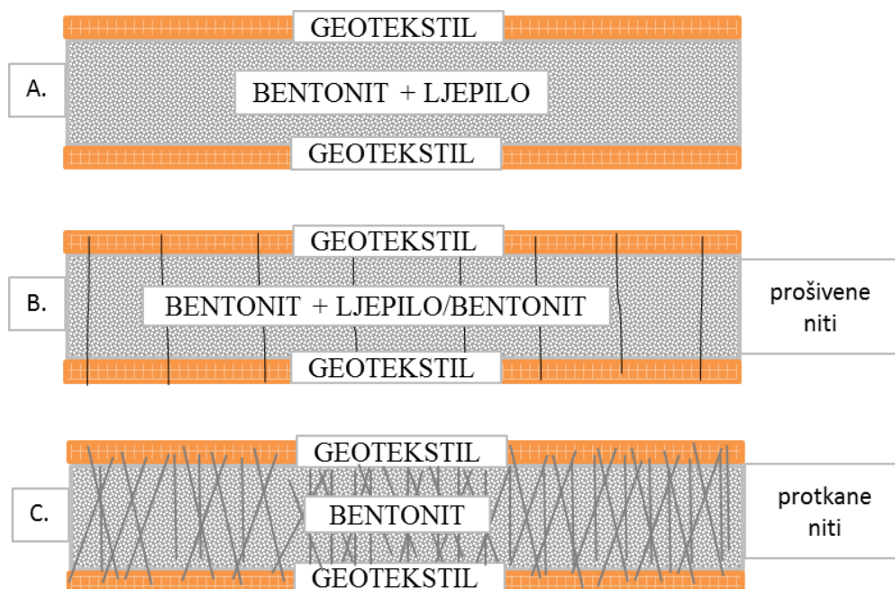
Slika 2-5. Spajanje bentonita i geotekstila
