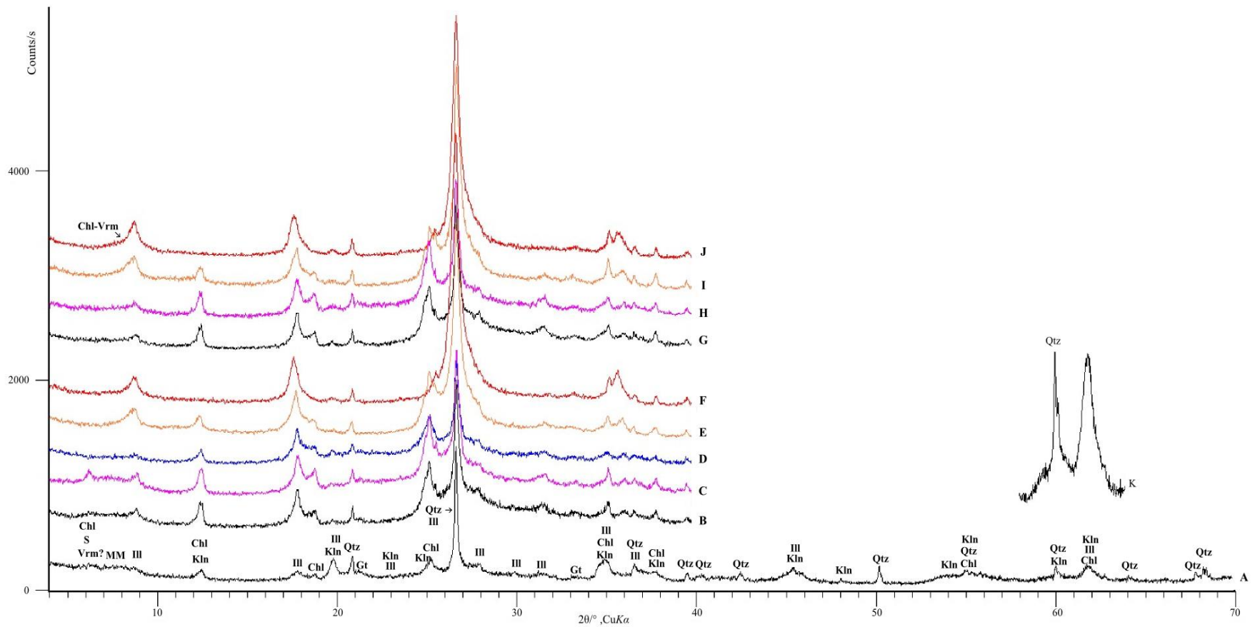
Slika 5-27. Difrakcijske slike glinovite frakcije uzorka 4892 ( A i K predstavljaju snimke neorijetiranih uzorkaka, a B – J snimke orijetiranih uzorkaka): A - netretirani uzorak, B - uzorak tretiran s K^+ , C - uzorak tretiran s K^+ saturiran s etilen-glikolom, D - uzorak tretiran s K^+ saturiran s dimetilsulfoksidom, E - uzorak tretiran s K^+ žaren na 350^\circ C , F - uzorak tretiran s K^+ žaren na 550^\circ C , G - uzorak tretiran s Mg^{2+} , H - uzorak tretiran s Mg^{2+} saturiran s etilen-glikolom, I - uzorak tretiran s Mg^{2+} žaren na 350^\circ C , J - uzorak tretiran s Mg^{2+} žaren na 550^\circ C ; K - difrakcijska linija 060. Tumač kratica: Qtz – kvarc, Chl – klorit, Ill – illitični materijal, Gt – getit, Kln – kaolinit, MM-miješanoslojni minerali glina, Vrm – vermikulit, S – smektit.
