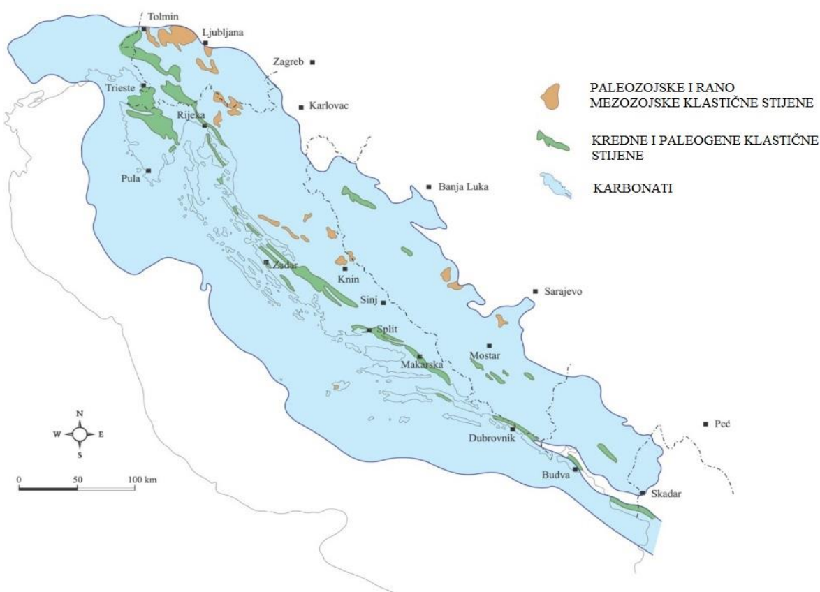
Slika 2.5. Sastav stijena Krških Dinarida (prema Velić et al., 2002).
