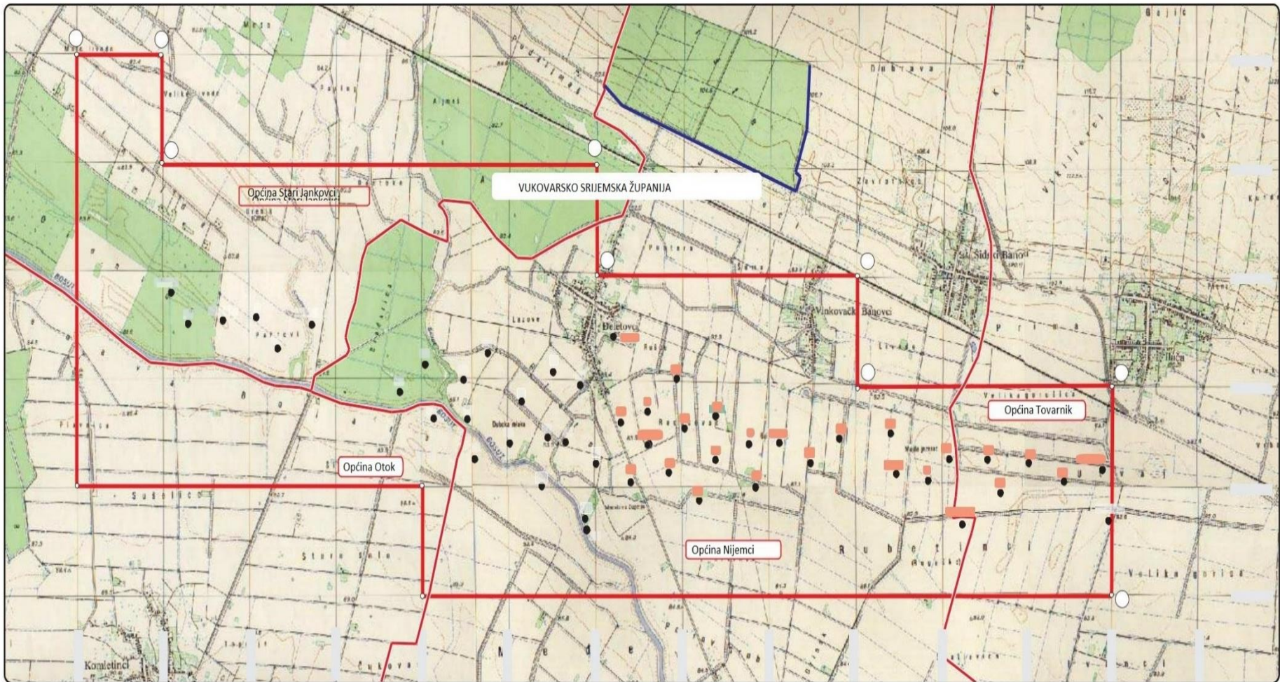
Slika 2.8. Eksploatacijsko polje Đeletovci s ucrtanim bušotinama i granicama.
