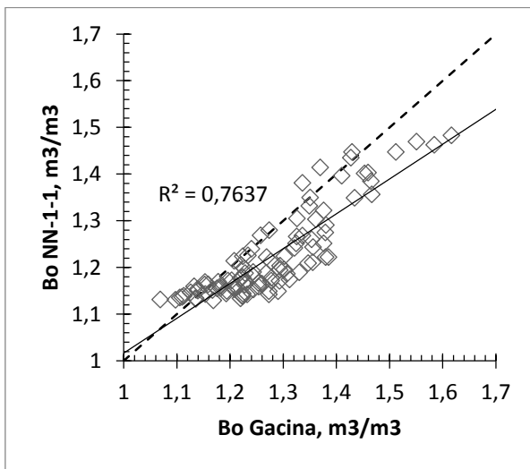
Slika 4-9 Volumni faktor nafte Gaćininom korelacijom i volumni faktor nafte neuronskom mrežom NN-1-1
