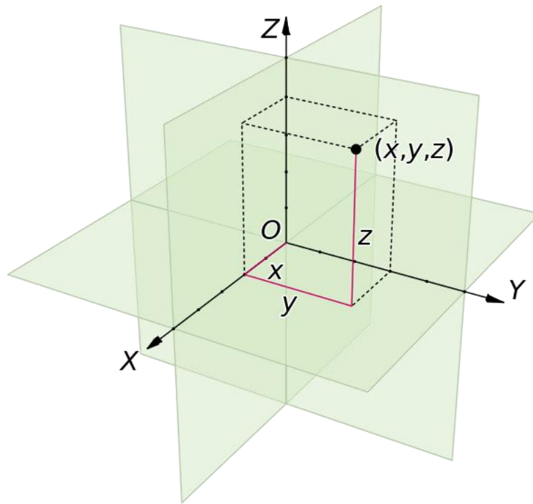
Slika 4.1. Kartezijev koordinatni sustav
