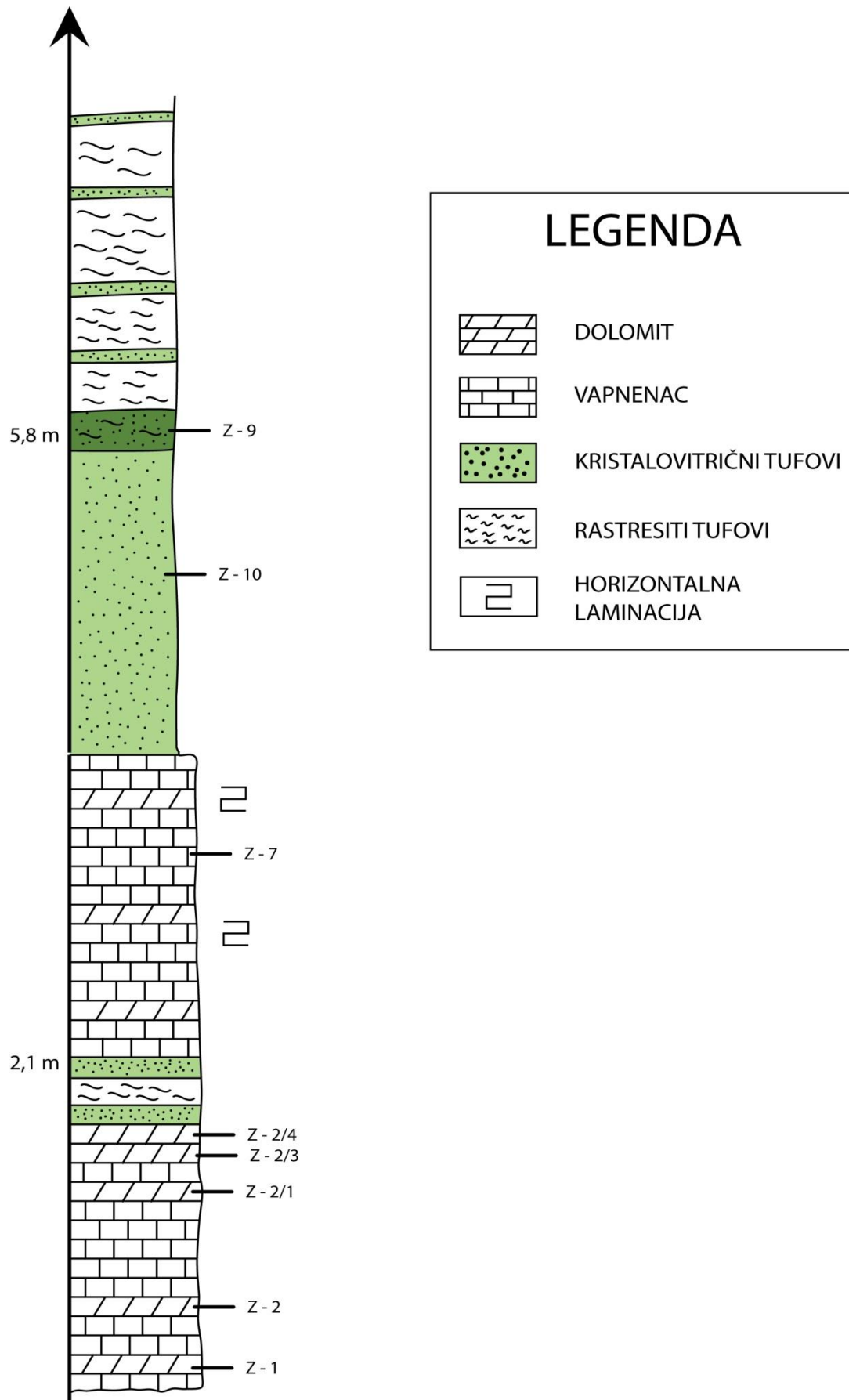
Slika 5.2.1. Slijed naslaga snimljen na lokalitetu ZELOVO ( "Z" )
