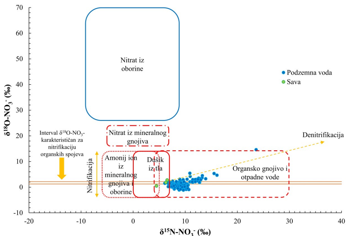
Slika 6.8. Prikaz \delta^{15}\text{N-NO}_3^- i \delta^{18}\text{O-NO}_3^- u svim uzorcima
