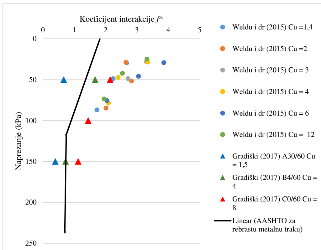
Slika 7-9 Usporedba koeficijena interakcije geosintetičke trake za različite koeficijente nejednoličnosti s podacima za rebrastu metalnu traku
