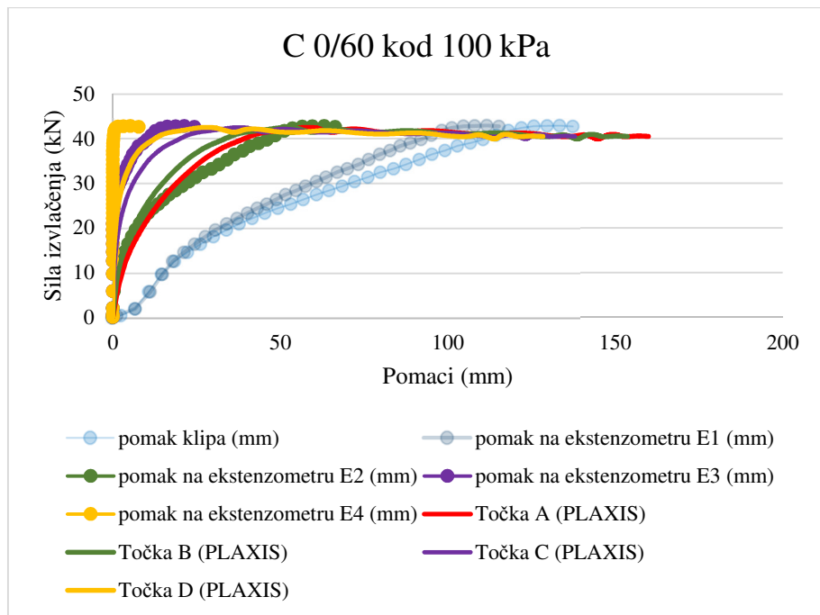
Slika 6-30 Razvoj sile izvlačenja po točkama u kojima su praćeni pomaci u laboratoriju i numerički za C0/60 kod 100 kPa
