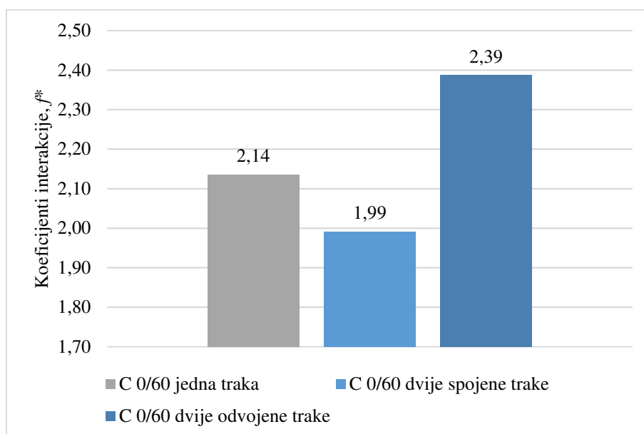
Slika 5-33 Usporedba koeficijenata interakcije za ispitivanje jedne trake, dvije spojene i dvije odvojene trake pri vertikalnom napreznju od 50 kPa
