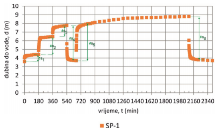
Slika 4.3. Dijagram kolebanja razine vode i prirasti sniženja ( \delta s_i ) za crpljnje u koracima pri pokusnom crpljenju (prema Hlevnjak i dr., 2014)
