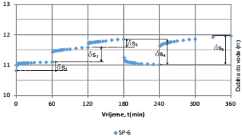
Slika 4.6. Dijagram kolebanja razine vode i prirasti sniženja ( \delta s_i ) za crpljnje u koracima pri pokusnom crpljenju. (prema Hlevnjak i dr., 2014)
