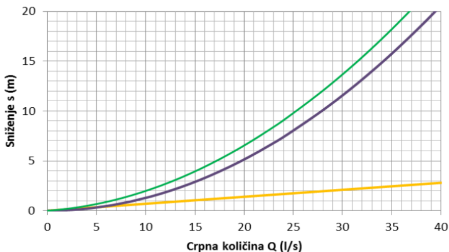
Slika 4.8. Dijagram s=f(Q) i pojedine vrste gubitaka za crpljenje bušotine SP-6. (prema Hlevnjaki dr., 2014)
