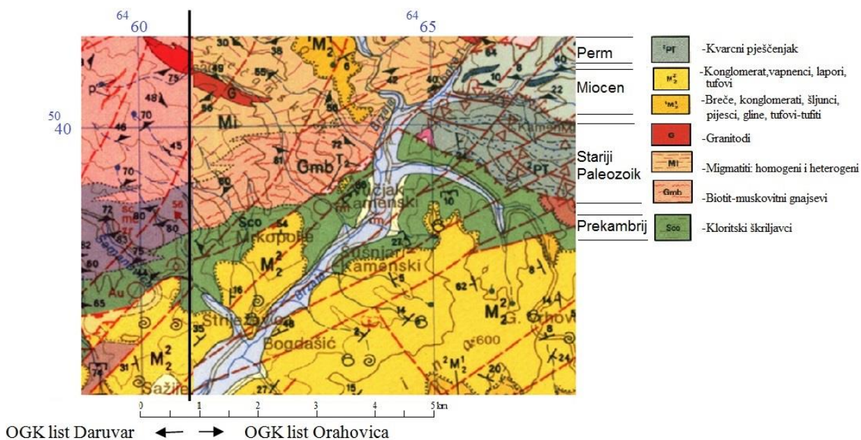
Slika 2.2 OGK Daruvara i Orahovice (prema Jamičić, D., Brkić, M. 1987)
