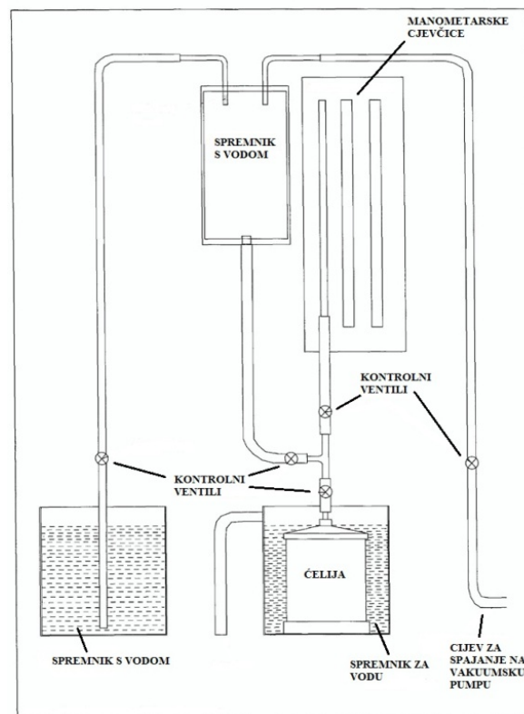
Slika 5.18. Skica rasporeda aparature prilikom izvođenja eksperimenta permeametrovom s promjenjivom razinom (ELE International, 2003).
