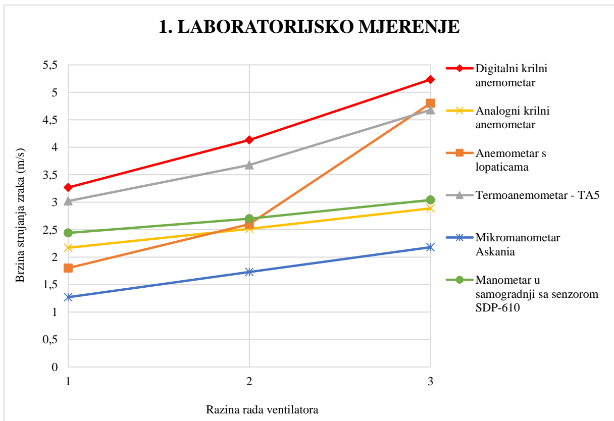
Slika 7-1. Dijagram odnosa brzine strujanja zraka i razine rada ventilatora kod različitih uređaja u cijevi promjera 110 mm.
