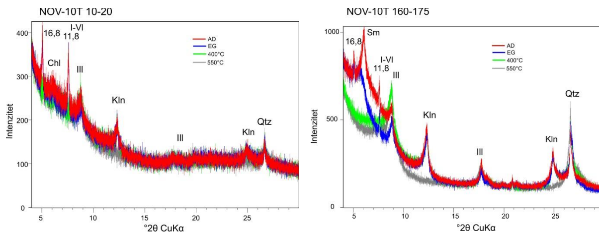
Prilog 76. Rendgenogrami orijentiranih preparata uzoraka iz jezgre NOV-10T. Oznake: AD-sušen na zraku, EG-tretiran s etilen glikolom, G-tretiran s glicerolom, DMSO-dimetil sulfoksidi, Ill-ilit, Kln-neuređen kaolinit, KlnD-uređen kaolinit, V-vermikulit, Qtz-kvarc, I-V-ilit-vermikulit.
