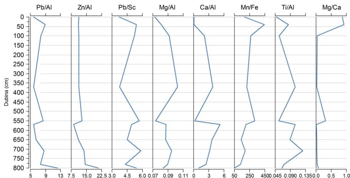
Slika 5.72. Raspodjela odabranih odnosa kemijskih elemenata (Pb/Al, Zn/Al, Pb/Sc, Mg/Al, Ca/Al, Mn/Fe, Ti/Al, Mg/Ca) u profilu NOV-11.
