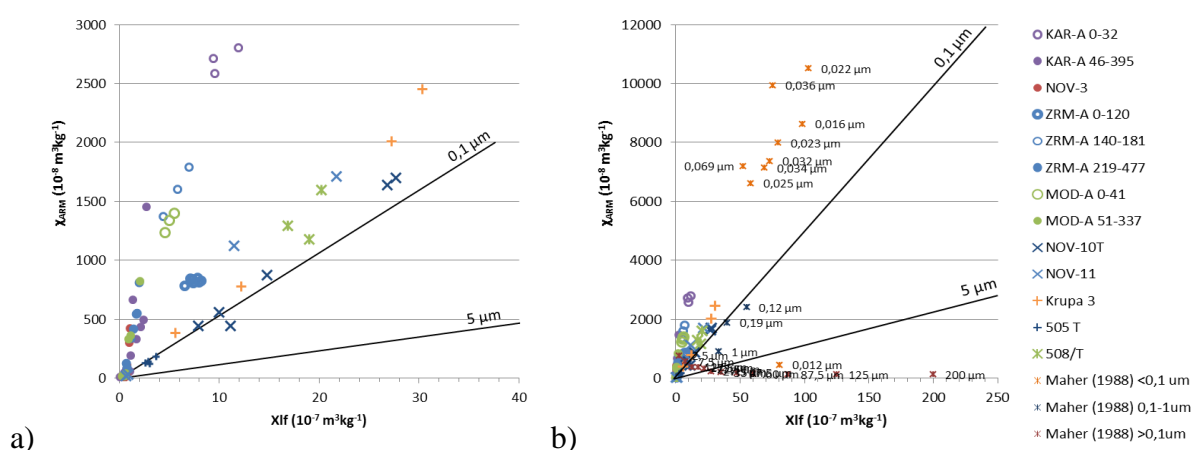
Slika 6.10. Graf \chi_{\text{ARM}}/\chi_{\text{IRM}} , tzv. „King plot“ korišten za razlikovanje veličine čestica (Banerjee et al., 1981, King et al., 1983). Odnos opada s porastom veličine magnetičnih čestica. Na grafu a) prikazani su rezultati mjerenja u ovom istraživanju, na grafu b) isti su pridruženi mjerenjima sintetskih magnetita (Maher, 1988).
