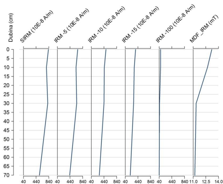
Slika 5.182. Vertikalna raspodjela \kappa_{lf} , \chi_{fd}(\%) , SIRM-a, demagnetizacije IRM-a pri vanjskom magnetskom polju od 5mT do 300mT i MDF_{IRM} -a u jezgri 505/T.
