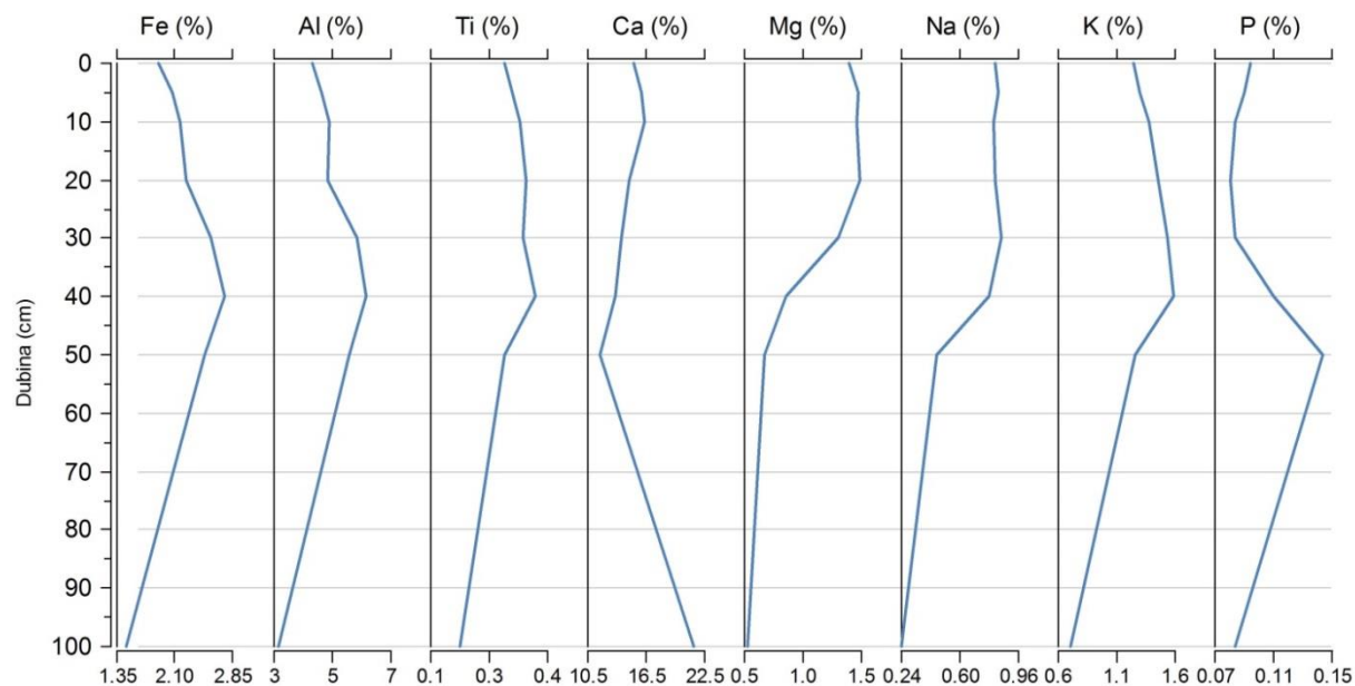
Slika 5.93. Raspođjela odabranih glavnih elemenata (Fe, Al, Ti, Ca, Mg, Na, K i P) u jezgri 509 F.
