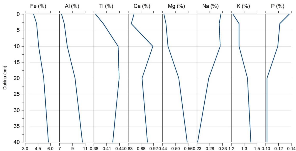
Slika 5.105. Raspodjela odabranih glavnih elemenata (Fe, Al, Ti, Ca, Mg, Na, K i P) u profilu Klanci.
