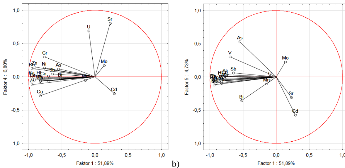
Slika 5.124. a) Dijagram ovisnosti Faktora 1 i Faktora 4 od 22 elementa morske jezgre NOV-3. b) Dijagram ovisnosti Faktora 1 i Faktora 5 od 22 elementa morske jezgre NOV-3.
