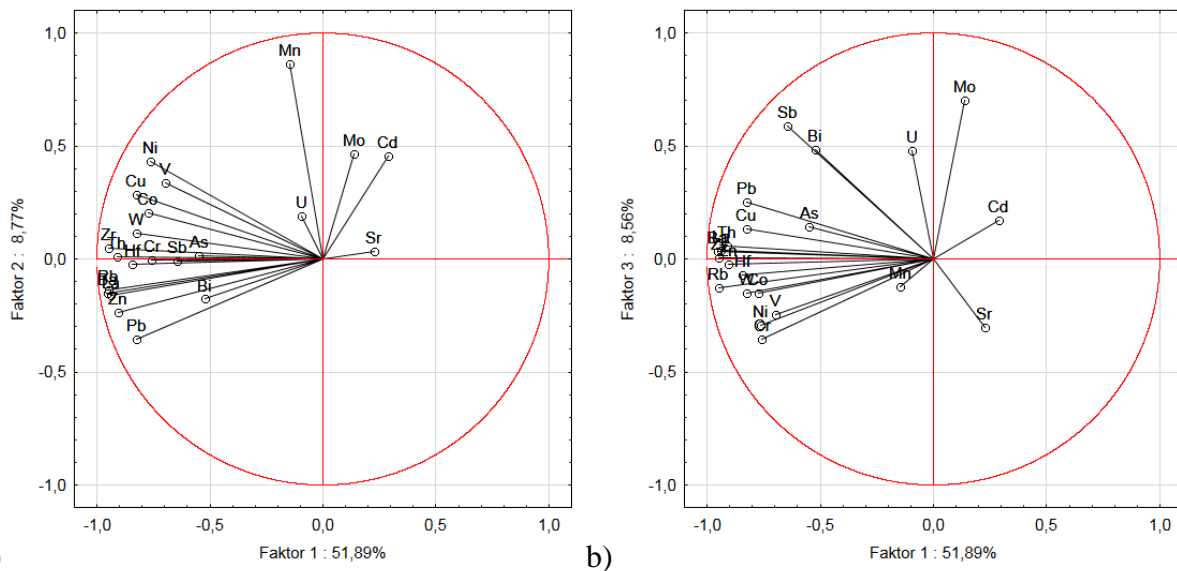
Slika 5.123. a) Dijagram ovisnosti Faktora 1 i Faktora 2 od 22 elementa morske jezgre NOV-3. b) Dijagram ovisnosti Faktora 1 i Faktora 3 od 22 elementa morske jezgre NOV-3.
