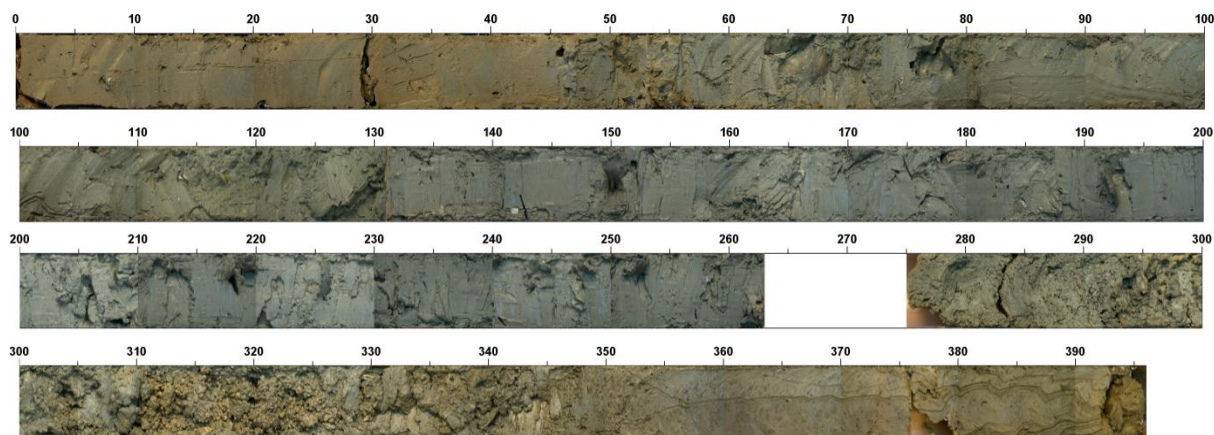
Slika 5.1. Digitalni snimak jezgre KAR-A prikazan u intervalima od 100 cm. Vidljiva je promjena boje od 10YR do 5Y. Također se ističe interval 275-350 cm koji je krupnozrnatiji i manje homogen.
