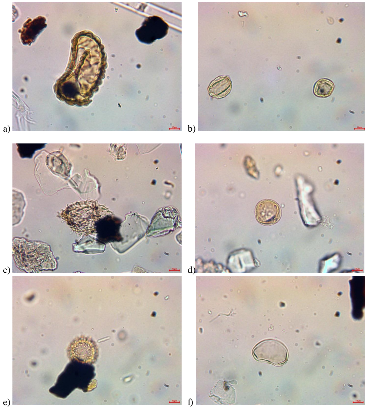
Prilog 122. Tipičan sastav palinomorfâ jezgre KAR-A. a) Polypodium (KAR-A 308-312 cm); b) Quercus (KAR-A 318-321 cm); c) ? Polyspheridium (KAR-A 338-342 cm); d) Pistacia (KAR-A 338-342 cm); e) cf. Nymphaea (KAR-A 353-357 cm); f) Polypodium (KAR-A 353-357 cm). Grafičko mjerilo (crvena linija u donjem desnom kutu) je veličine 10 \mu\text{m} .
