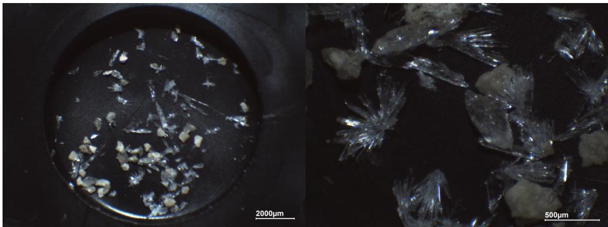
Prilog 94. Kristali gipsa u uzorku KAR-A 321-323.
