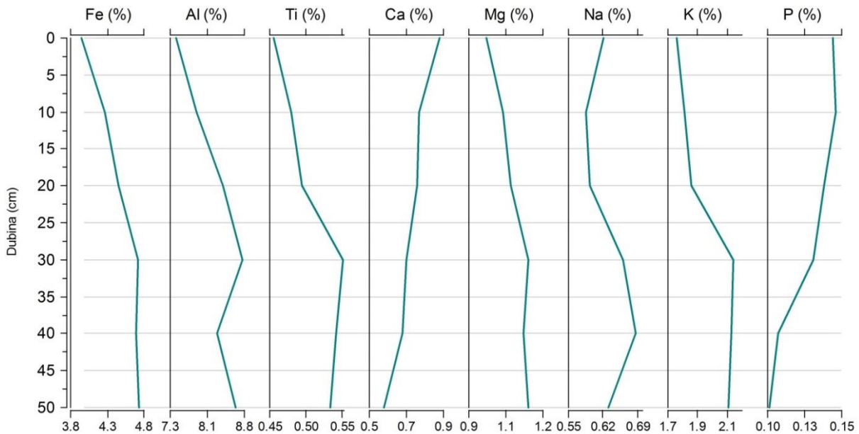
Slika 5.101. Raspodjela odabranih glavnih elemenata (Fe, Al, Ti, Ca, Mg, Na, K i P) u profilu Crnopac.
