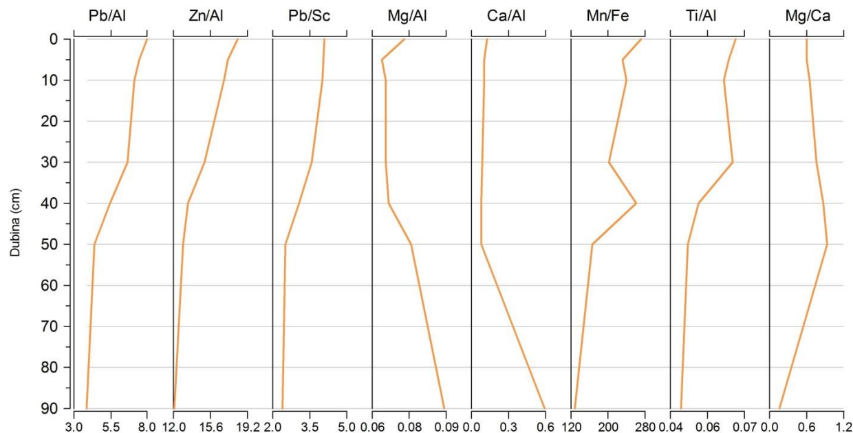
Slika 5.80. Raspodjela odabranih odnosa kemijskih elemenata (Pb/Al, Zn/Al, Pb/Sc, Mg/Al, Ca/Al, Mn/Fe, Ti/Al, Mg/Ca) u jezgri 505F.
