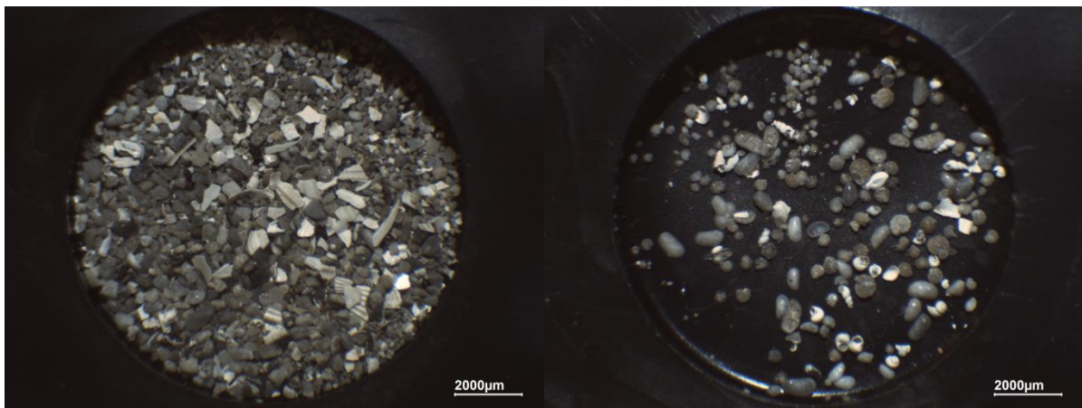
Prilog 107. Ukupni (lijevo) i fosilni (desno) sadržaj uzorka NOV-3 600-602.
