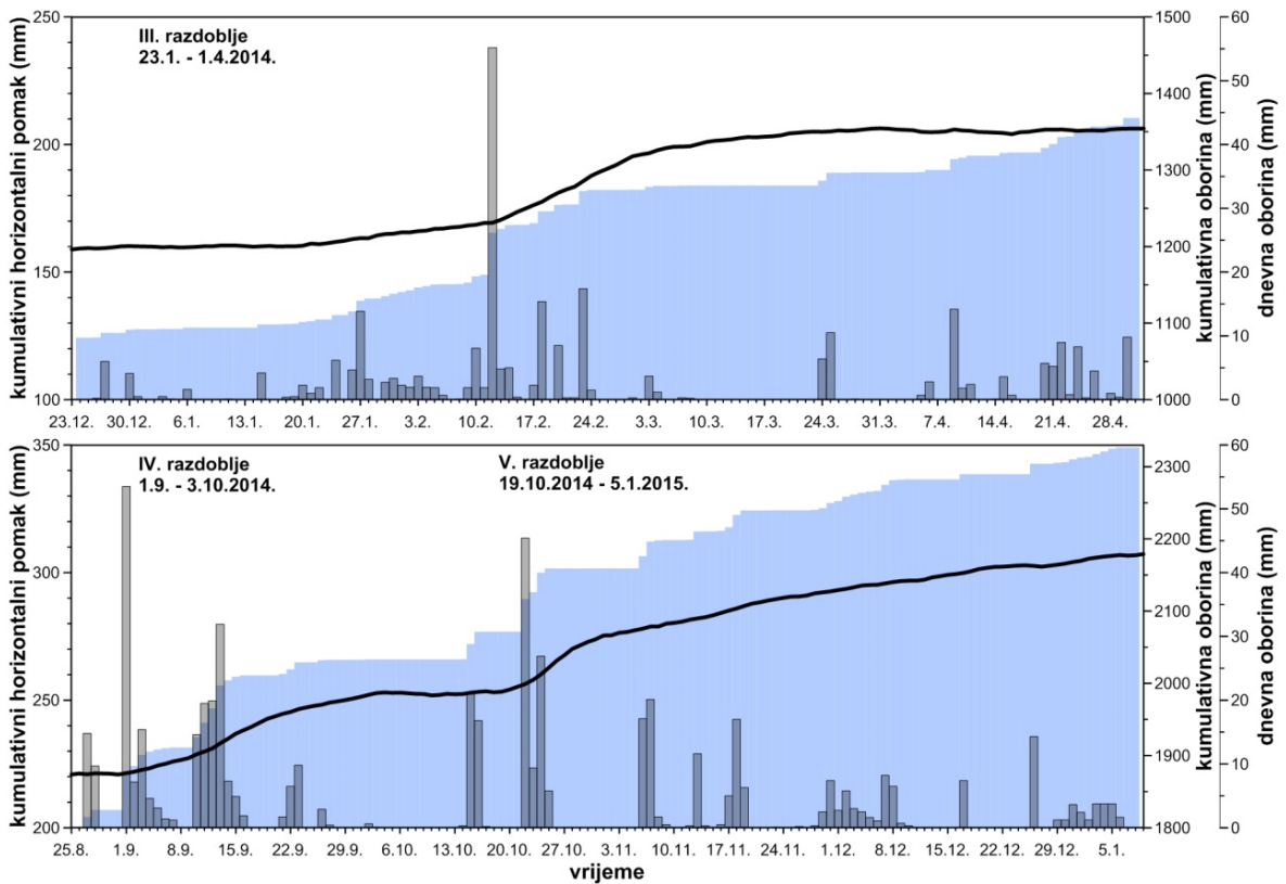
Slika 6.43. Kumulativni horizontalni pomaci, dnevne oborine i kumulativne dnevne oborine u razdobljima bržeg gibnja III, IV i V.
