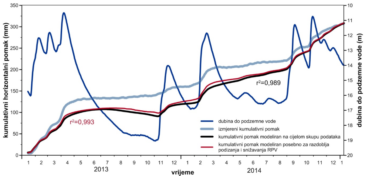
Slika 6.35. Odnos između izmjerenog kumulativnog horizontalnog pomaka klizišta i pomaka klizišta određenih na temelju brzina modeliranih višestrukim linearnom regresijom.
