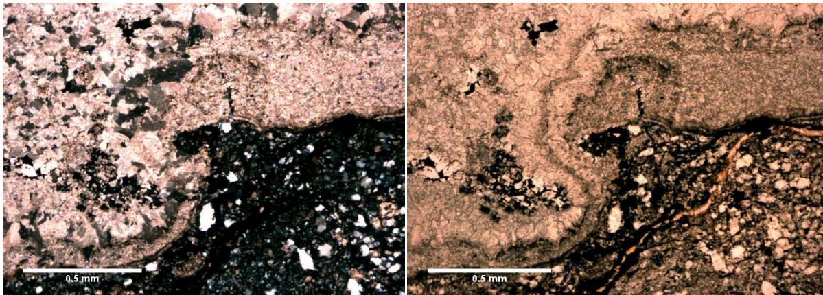
Slika 5.23 Mikrofotografije uzorka ID 7 KONTAKT DOLOMITA i PJEŠČENJAKA; a - s analizatorom, b –bez analizatora
